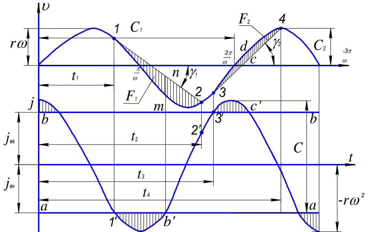
Рисунок 2. Графики скоростей и ускорений решетчатого стана и зернового материала
