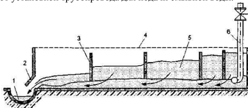
Рисунок 2.3 - Секционная система навозоудаления периодического действия: 1 - поперечный коллектор; 2 - шиберное устройство; 3 - неподвижная поперечная перегородка; 4 - щелевой пол; 5 - навозоприемный лоток — поперечный канал; 6 - смывной трубопровод с задвижкой
