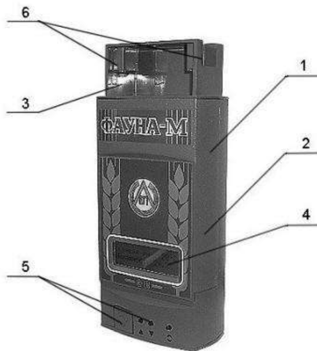
Рисунок 5.1.- Общий вид влагомера Фауна-ВЛК:
