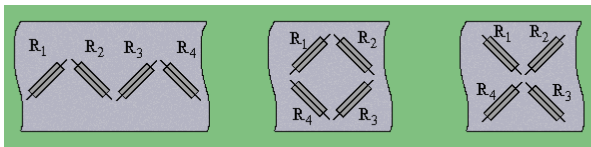
Рисунок 7.5.- Схемы наклейки тензорезисторов для измерения крутящего момента.
