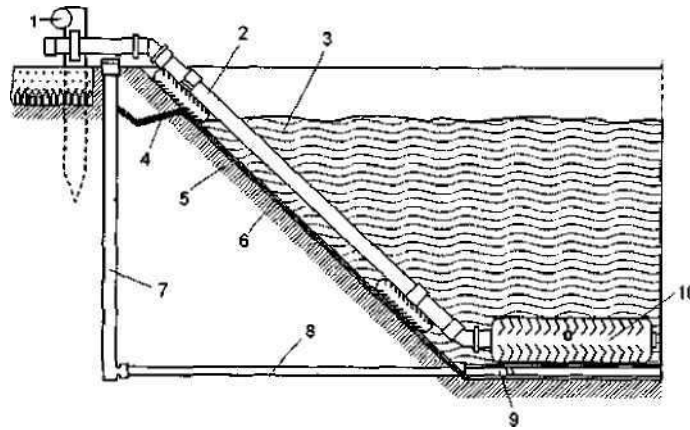
Рисунок 4.5 - Схема накопителя навоза с пленочным экраном: 1 - ограждающий барьер; 2 - трубопровод для навоза; 3 - уровень навоза; 4— гидроизоляционная пленка; 5—глинистый экран; 6—тонкая полимерная пленка; 7— контрольная труба; 8—труба дренажной системы; 9—отверстие в трубе; 10—старая крышка, заполненная бетоном
