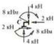
Рисунок 3.9 - Узел С
