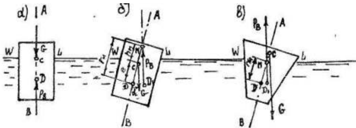
Рисунок 1-5. К расчету плавания тел:
