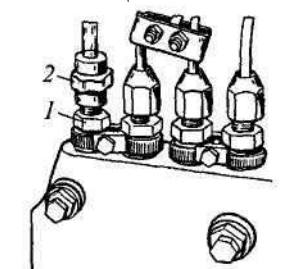
1 - штуцер топливного насоса; 2 - моментоскоп
