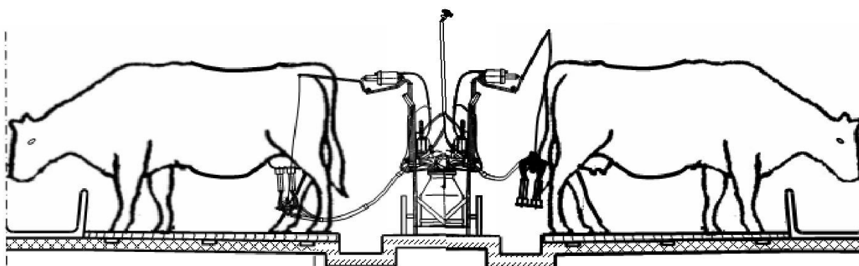
Рисунок 20– Технологическая схема работы мобильного доильного модуля в стойлах коровников при доении коров в два ряда.
