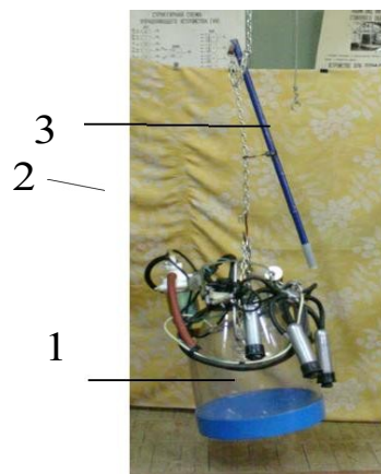
1 – доильное ведро; 2 – подвеска (цепь); 3 – рычаг
