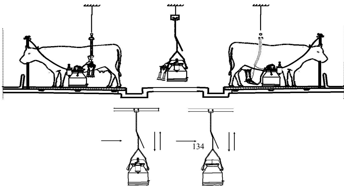
Рисунок 24 – Доильное ведро на подвеске, снабженное рычагом.
