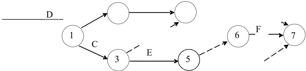
Рис. Сетевой график проекта
