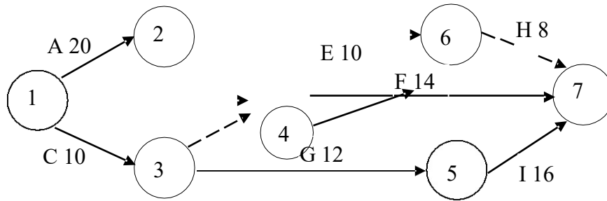
Рис. Сетевая модель проекта
