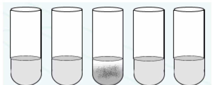
Рисунок 74 - Реакция флокуляции.
