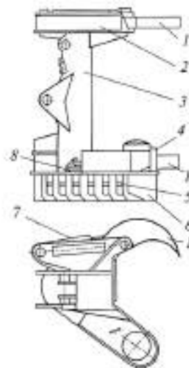
Рис. 3.5. Захватно-срезающее устройство: 1 — зажимные крюки; 2, 4 — соответственно верхняя и нижняя призмы; 3 — стойка; 5 — механизм среза; 6 — рама пилы; 7 — гидроцилиндр; 8 — трубопровод
