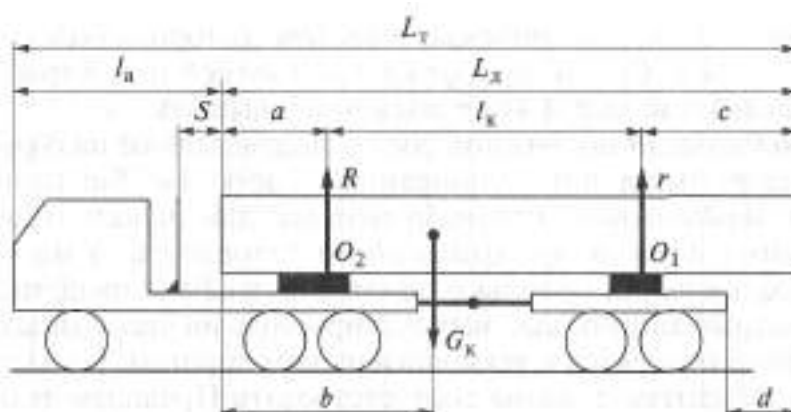
Рис. 4.4. Схема автопоезда к расчету расстояния между кониками: l_a — длина транспортного средства; L_x — длина деревьев или хлыстов; S — расстояние безопасности между пачкой хлыстов и защитной решеткой; c — расстояние от коника роспуска до крайней задней точки транспортного средства; d — свес груза
