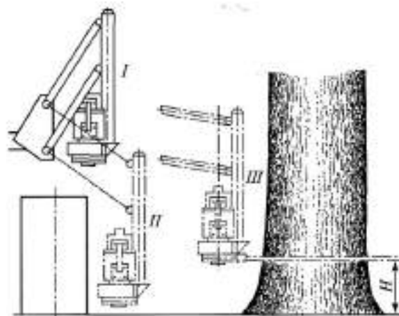
Рис. 1.3. Положение вертикальной наводки механизма срезания
