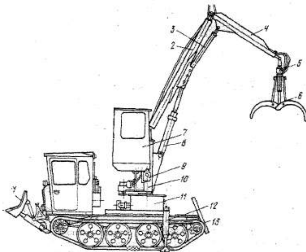
Рис. 4. Погрузчик-штабелер ПШ-80:
