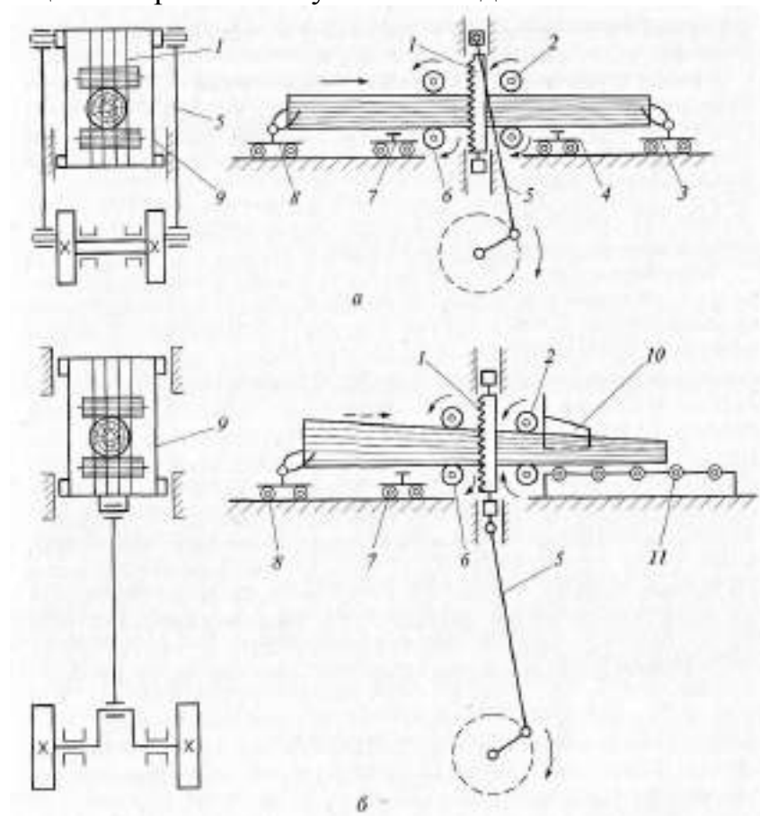
Рис. 6. Схемы двухштанной (а) и одноштанной (б) лесопильных рам:
