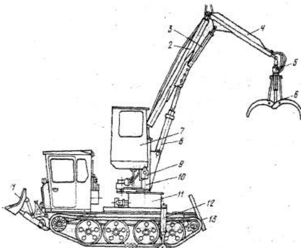
Рис. 4. Погрузчик-штабелер ПШ-80:
