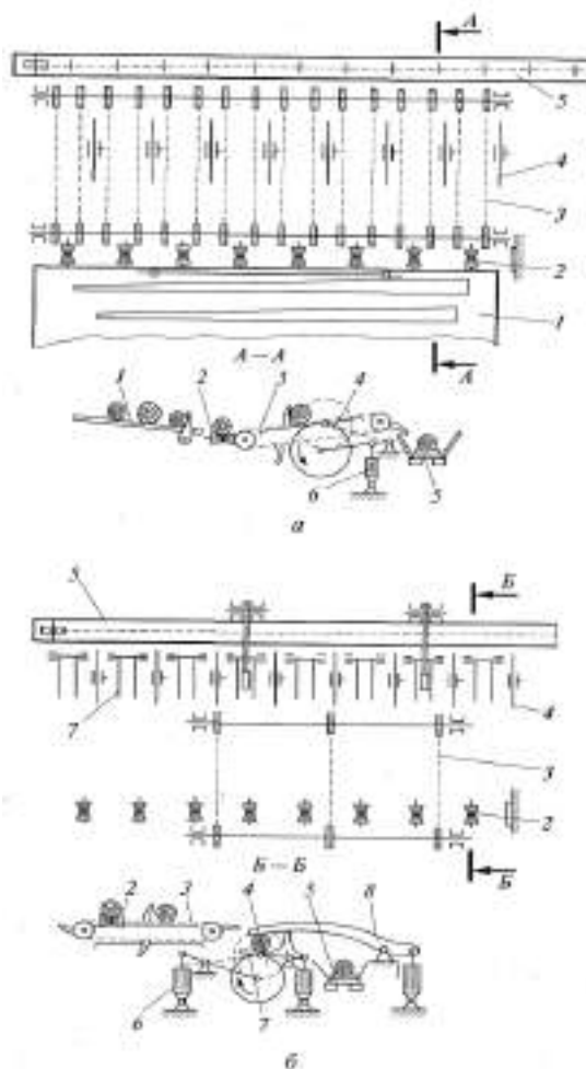
Рис. 3. Раскряжевочные установки с поперечным перемещением хлыста: а — триммер с непрерывным движением хлыста; б — триммер с пилением неподвижного хлыста; 7 — площадка; 2 — рольганг; 3 — поперечный транспортер; 4 — пила; 5 — выносной транспортер; 6 — индивидуальный привод пилы; 7 — сбрасыватель; 8 — рычаг
