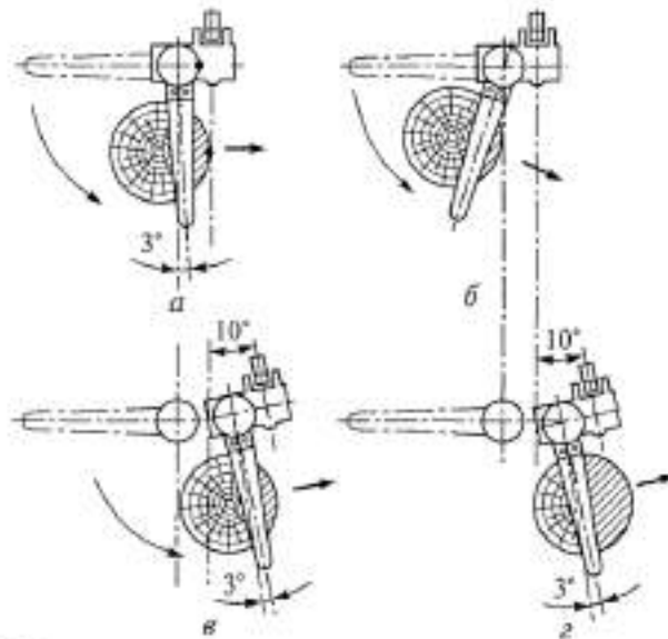
Рис. 1.5. Горизонтальная наводка механизма срезания на дерево: a — при валке дерева параллельно стенке леса; б — при валке без перекидывания дерева; в, г — при валке с перекидыванием дерева
