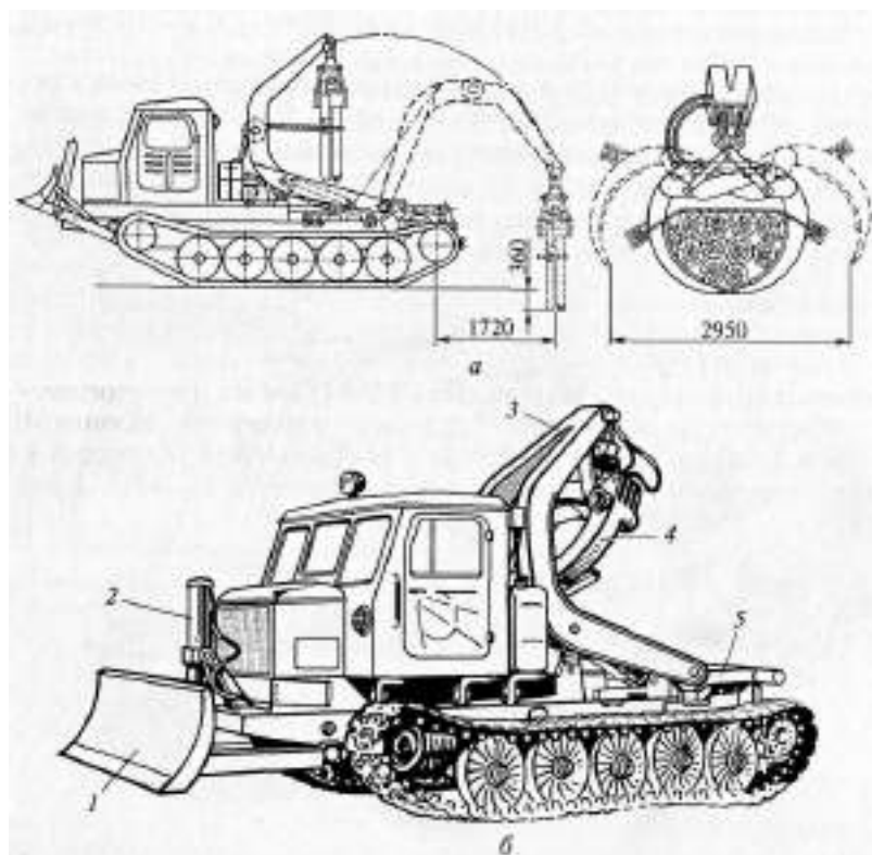
Рис. 7. Технологическое оборудование трактора ЛТ-154: a — схема работы; б — общий вид; 1 — толкатель; 2 — гидроцилиндр; 3 — стрела; 4 — клещевой пачковый захват; 5 — щит
