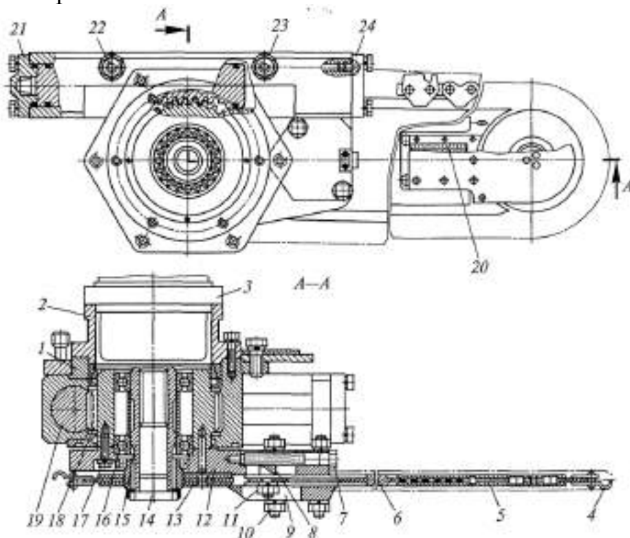
Рис. 3.6. Механизм срезания:
