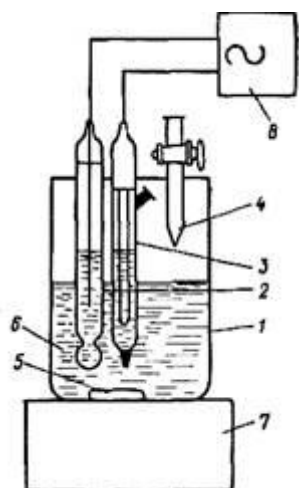
Рис. 3. Схема электрохимической ячейки для потенциометрического титрования 1 – химический стеклянный стакан; 2 – исследуемый раствор; 3 – хлорсеребряный электрод сравнения; 4 – бюретка со стандартным раствором; 5 – стеклянный индикаторный электрод; 6 – магнитная мешалка; 7 – магнитная мешалка; 8 – рН-метр.
