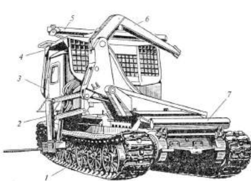
Рис. 3.1. Валочная машина ВМ-4:
