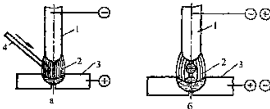
Рисунок 11.1. Схемы сварки неплавящимся (а) и плавящимся (б) электродами
