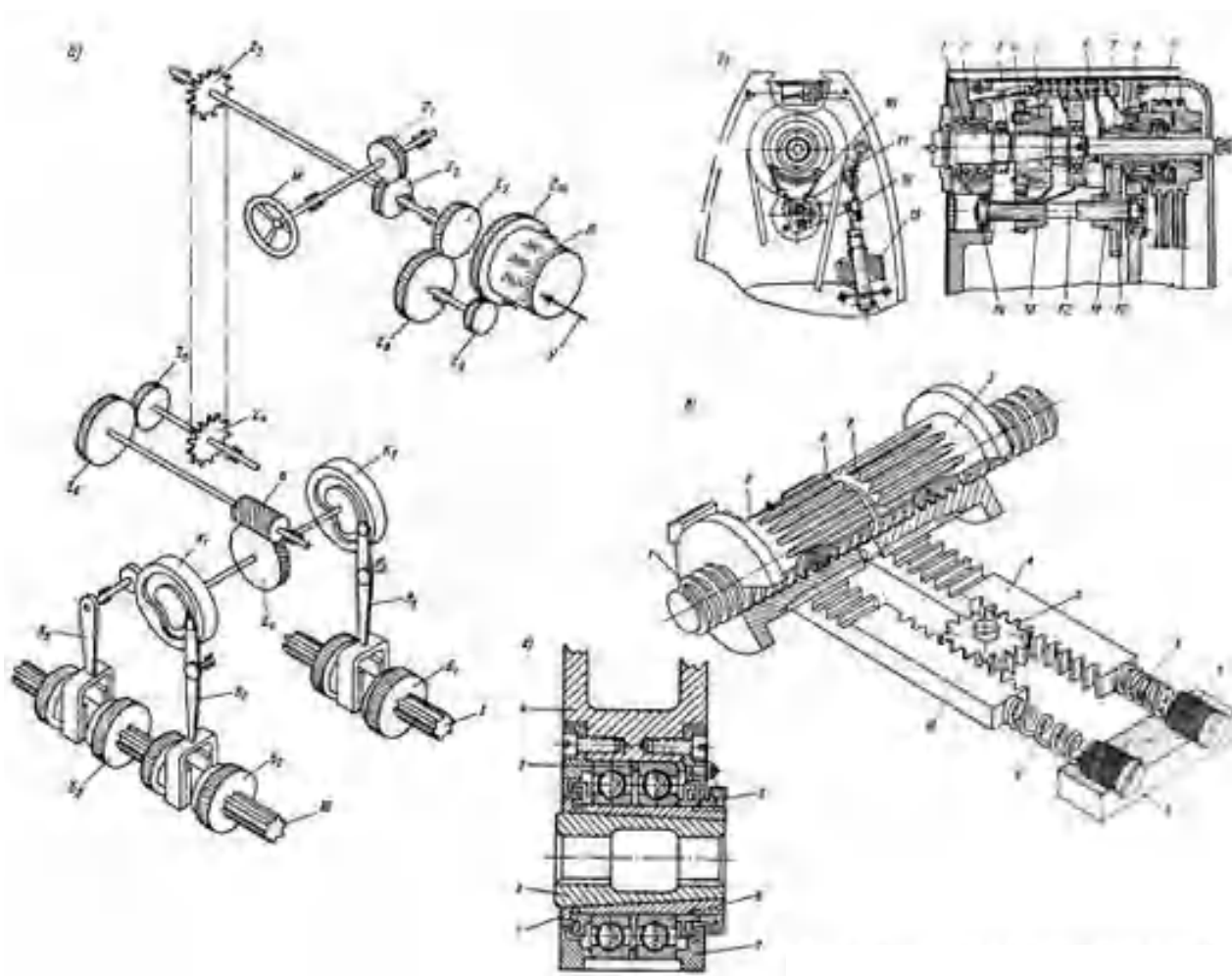
Рисунок 16.3. Узлы консольно-фрезерного станка 6Н81Г
