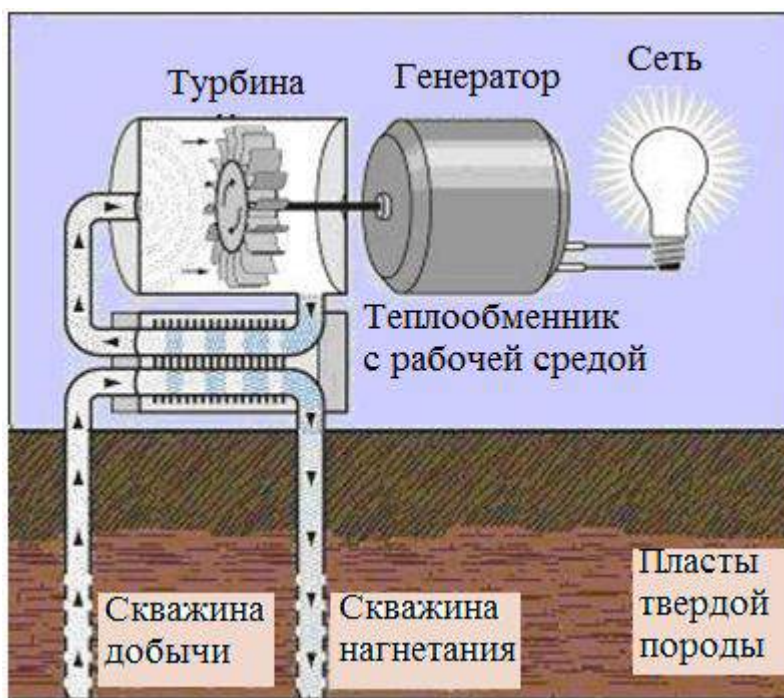
Рисунок 3 - Принцип работы геотермальной электростанции с бинарным циклом
