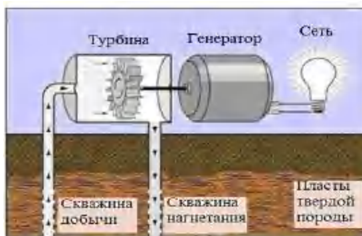
Рисунок 1 - Принцип работы геотермальной электростанции, работающей на сухом пару
