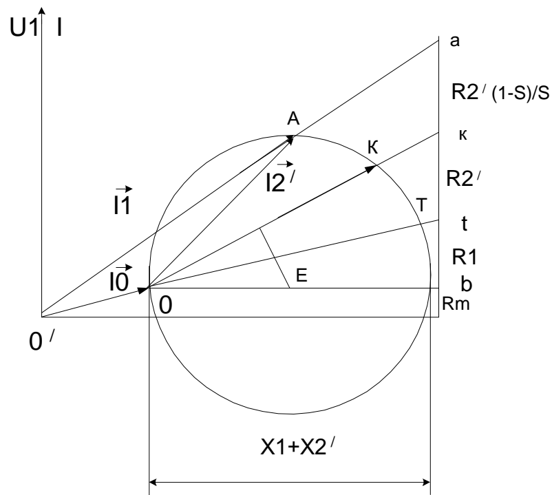
Рис.15.2. Круговая диаграмма АЭД.
