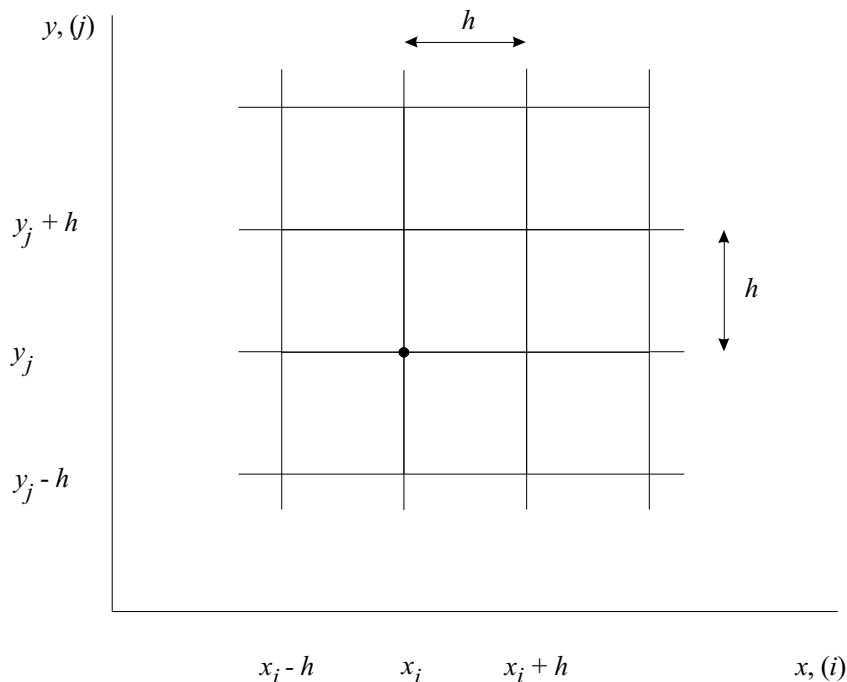
Рис. 3.2. Двумерная сетка
