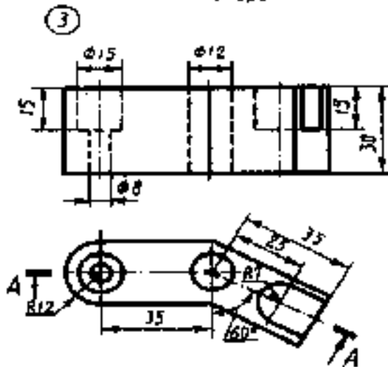
Скоба
