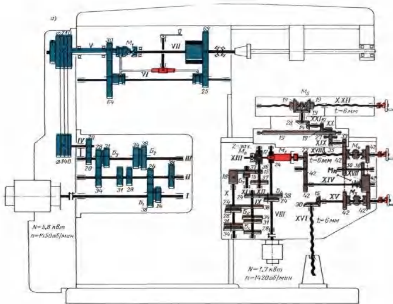
Рисунок 16.5. Схема кинематическая консольно-фрезерного станка 6Н81Г.
