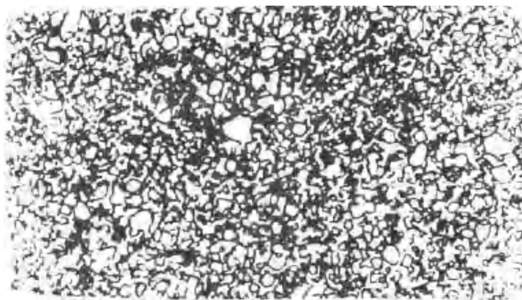
Рисунок 8.3. Микроструктура зернистого перлита x500
