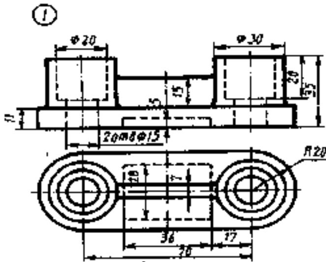
Опора
