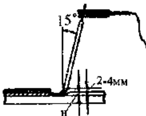
Рисунок 11.7. Положение электрода при сварке
