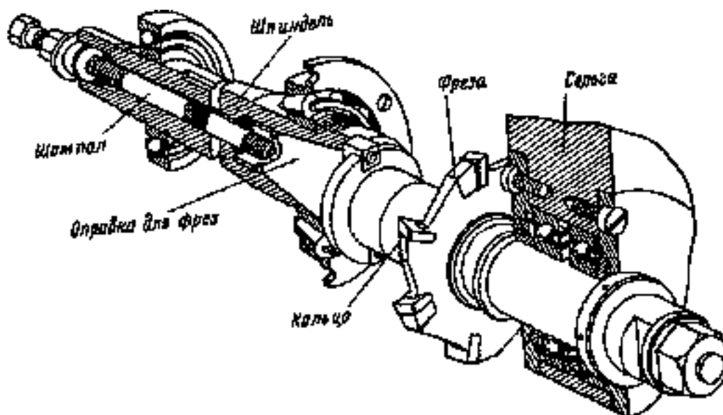
Рисунок 16.4. Установка инструмента на консольно-фрезерных станках 6Н81Г
