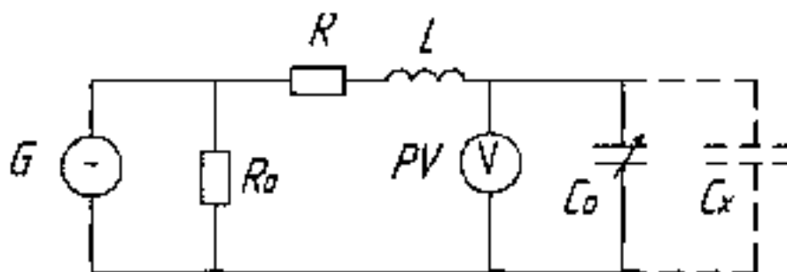
Рисунок 19.1. Принципиальная схема измерения емкости резонансным методом с вариацией реактивной проводимости
