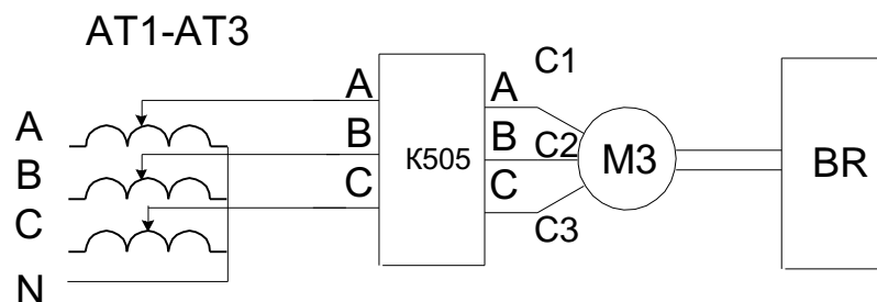
Рис.16.2. Схема включения асинхронного электродвигателя с короткозамкнутым ротором.
