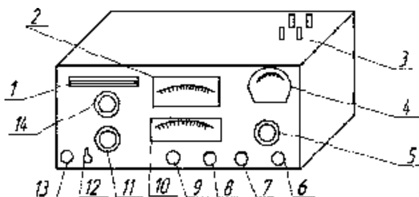
Рисунок 19.2. Измеритель добротности Е9-4 (ИДВ):
