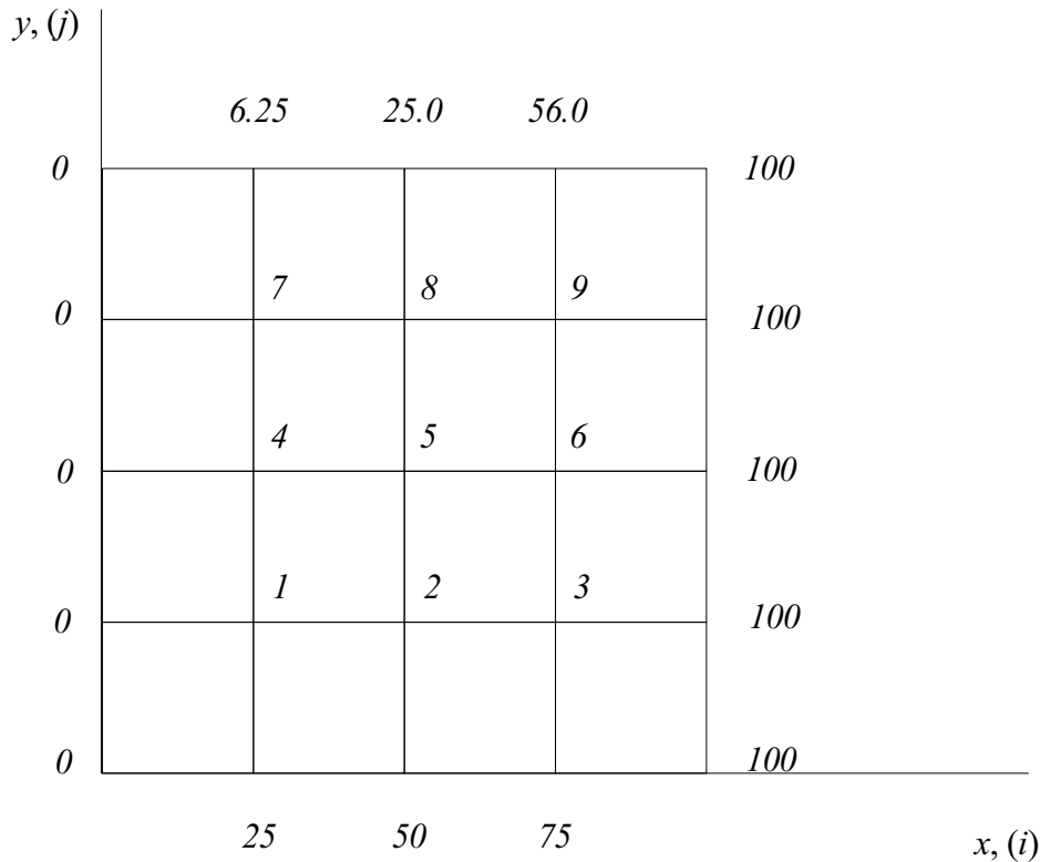
Рис. 3.3. Двумерная сетка и граничные условия
