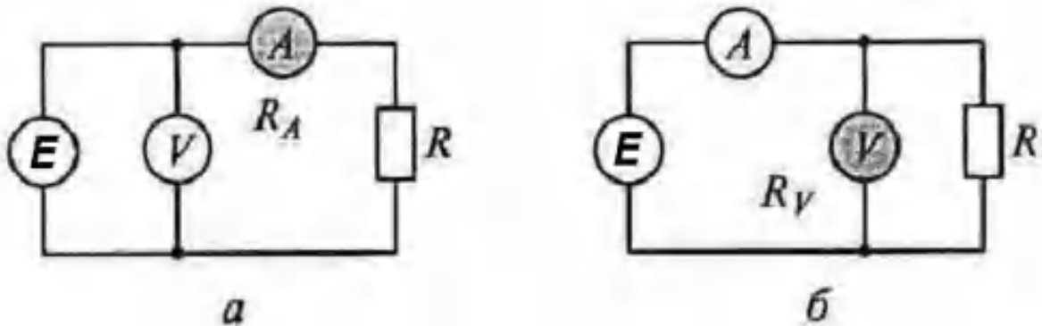
Рис. 1. Возникновение методической погрешности при различном подключении приборов: a — вольтметр—амперметр; b — амперметр—вольтметр
