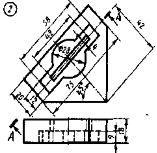
Пластина
