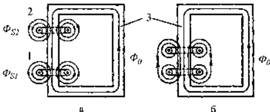
Рисунок 11.6. Схема магнитных потоков \Phi_{S1} и \Phi_{S2} сварочного трансформатора ТДМ при удалении (а) и сближении (б) вторичной (2) и первичной (1) обмоток
