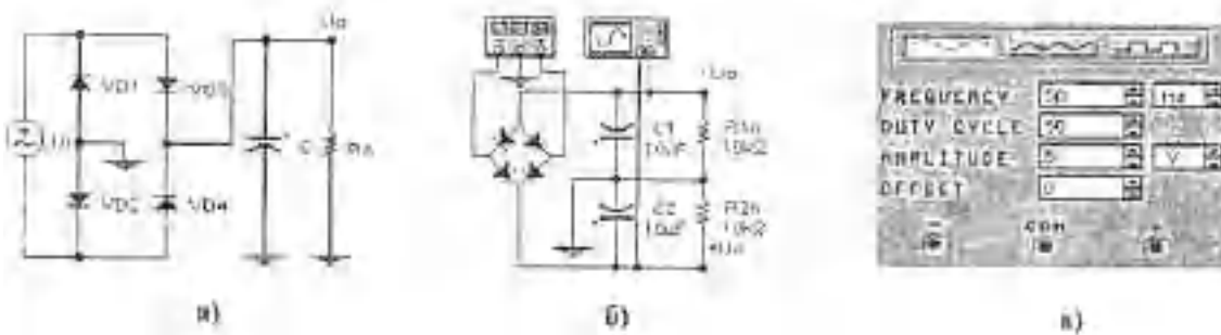
Рис. 2. Мостовые выпрямители
