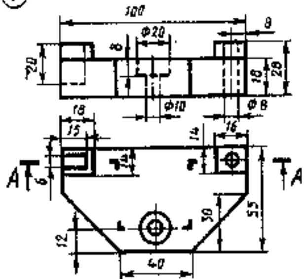
Пластина
