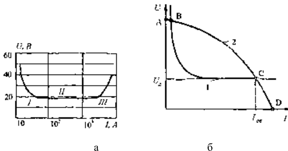
Рисунок 11.4. Вольтамперная характеристика дуги (а) и совмещенная вольтамперная характеристика дуги и источника тока (б)
