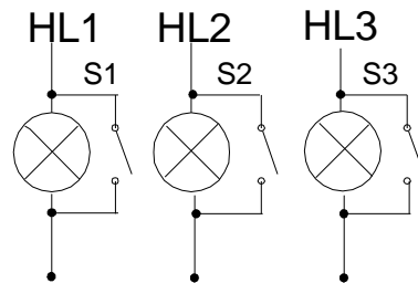
Рис.13.3 . Схема лампового синхроскопа.
