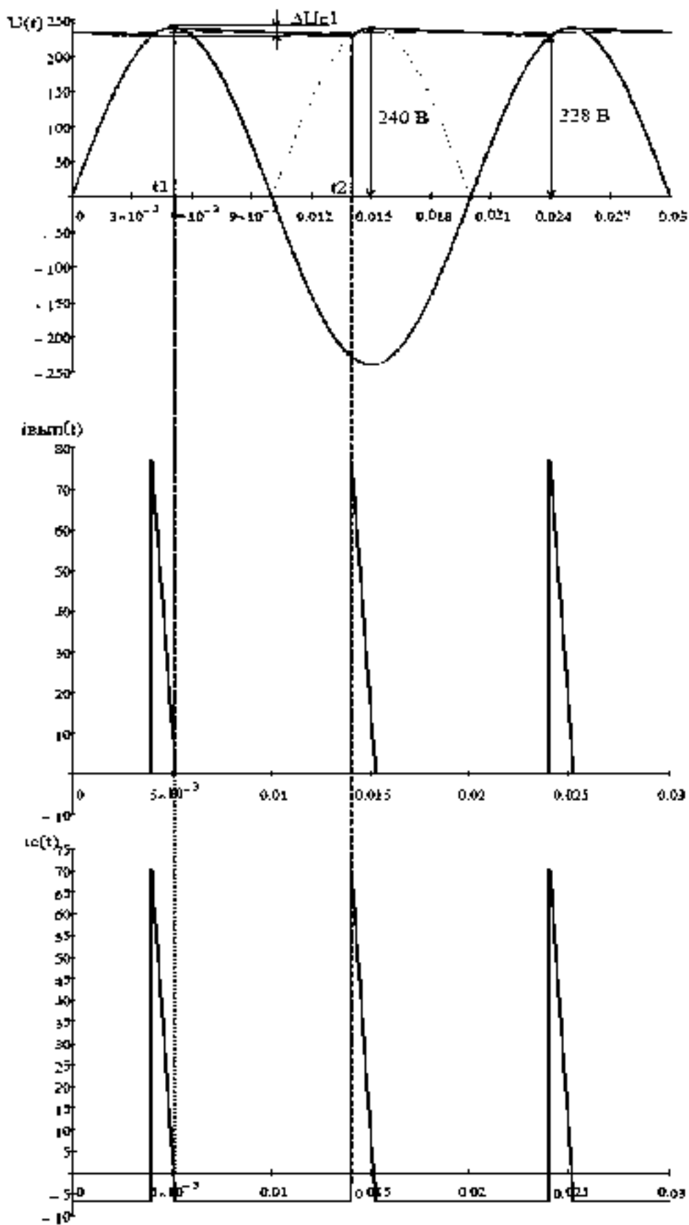
Рисунок 4 - Диаграммы токов и напряжений
