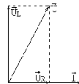
Рис. 1 Векторная диаграмма тока и напряжений
