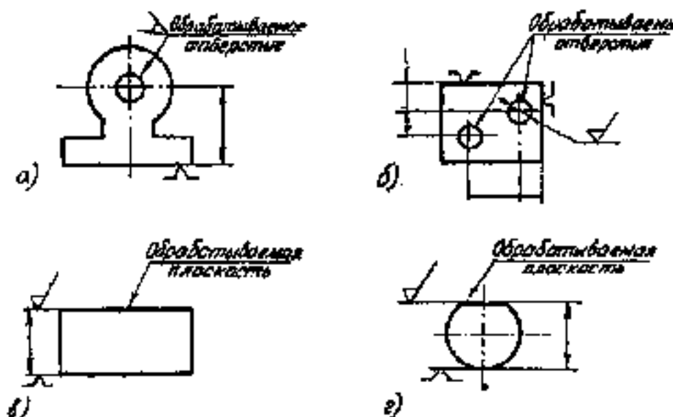
Рисунок 17.1. Схемы установки и базирования деталей
