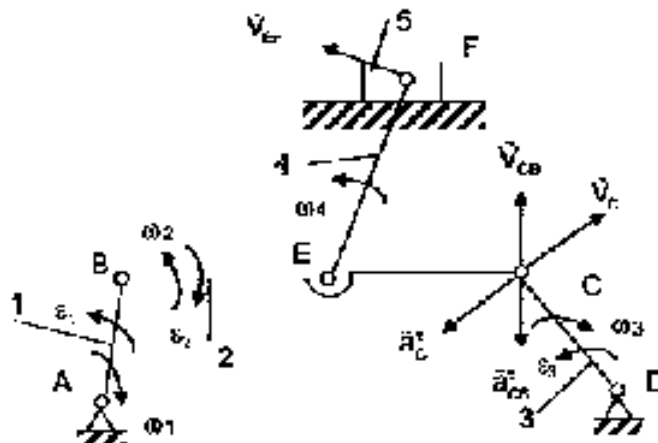
План скоростей
