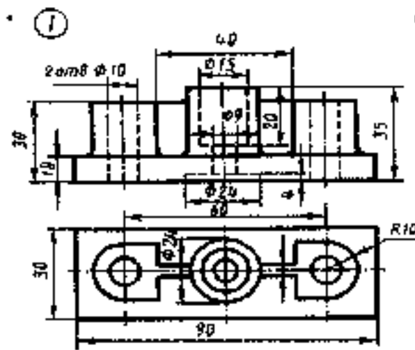
Корпус
