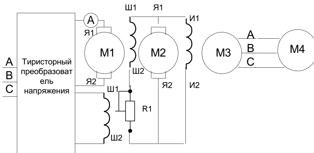
Рис.16.5. Схема включения асинхронного электродвигателя с короткозамкнутым ротором при частотном регулировании.
