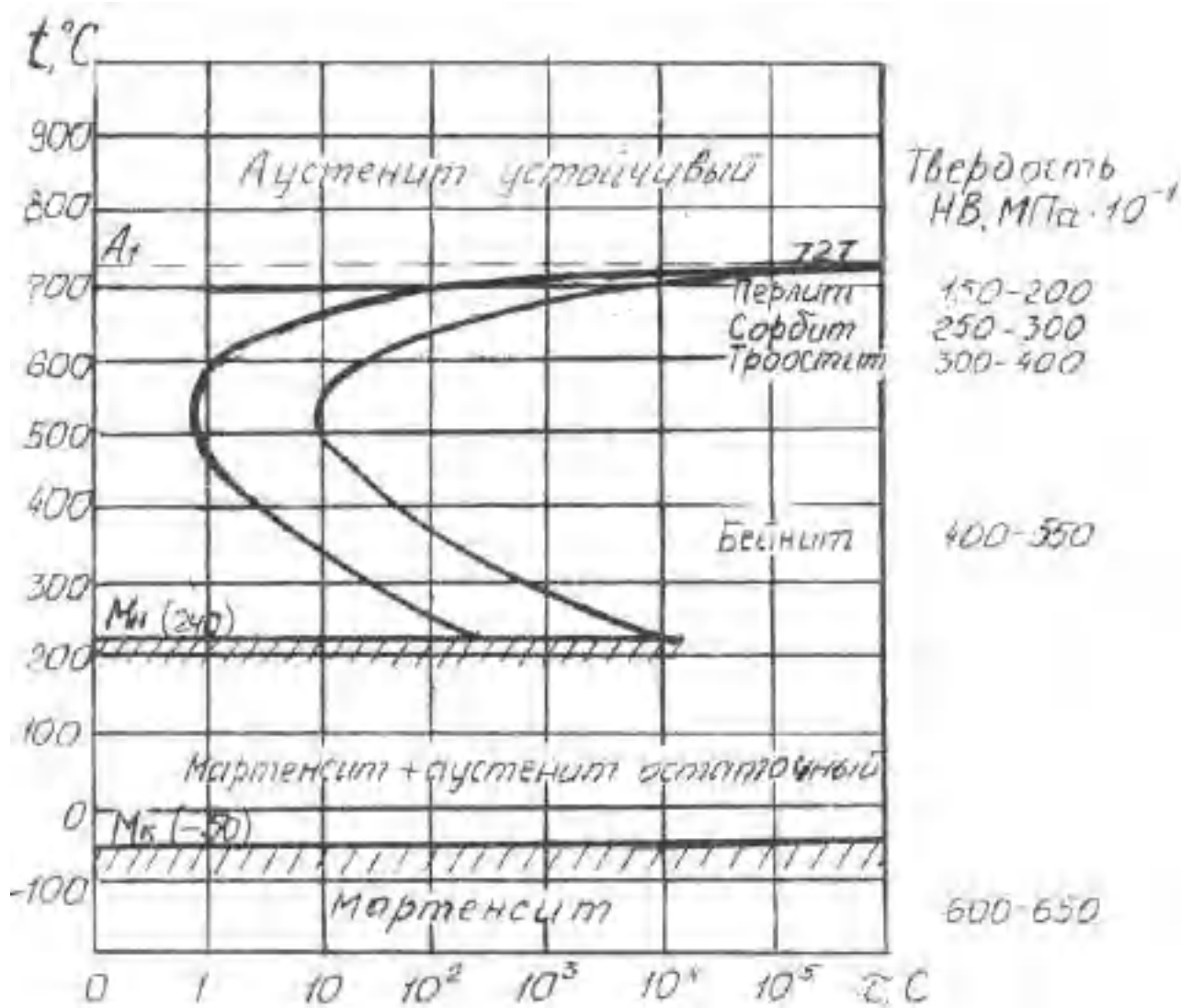
Рисунок 8.1. Диаграмма изотермического превращения аустенита эвтектоидной стали У8
