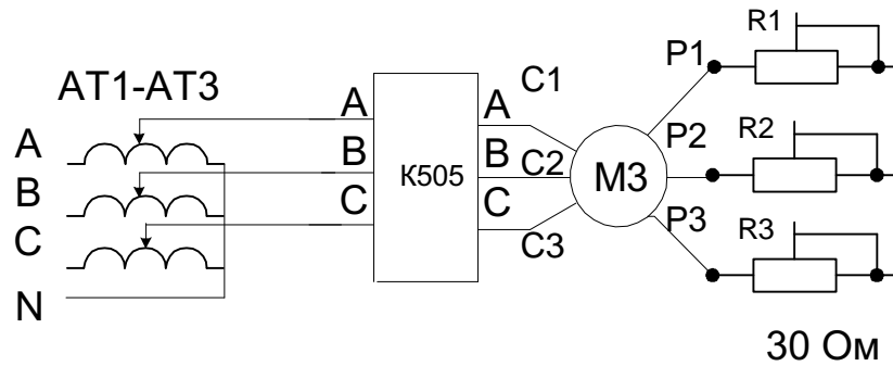
Рис.16.3. Схема включения асинхронного электродвигателя с фазным ротором при регулировании напряжением и роторными сопротивлениями.
