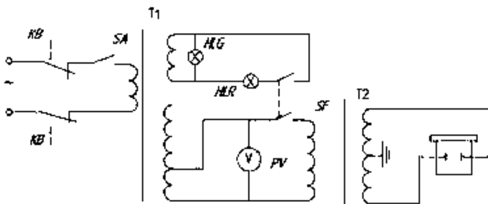
Рисунок 21.1. Электрическая схема аппарата АМИ-60
