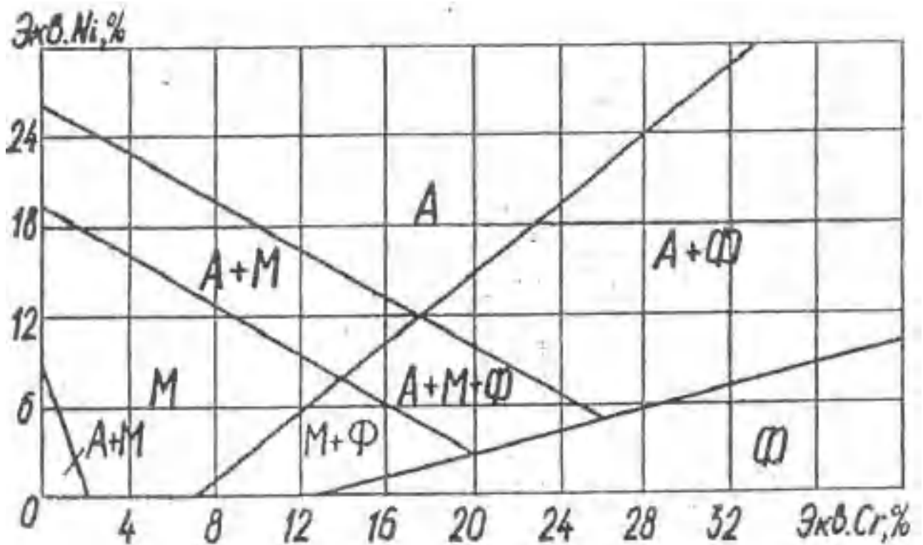
Рисунок 9.1. Структурная диаграмма коррозионностойких сталей (диаграмма Шеффлера)
