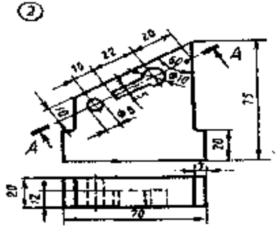
Ступка
