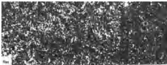
Рисунок 8.5. Микроструктуре троостита отпуска x500
