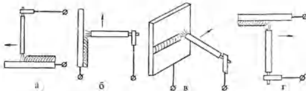
Рисунок 11.2. Возможные пространственные положения шва при ручной электродуговой сварке:
