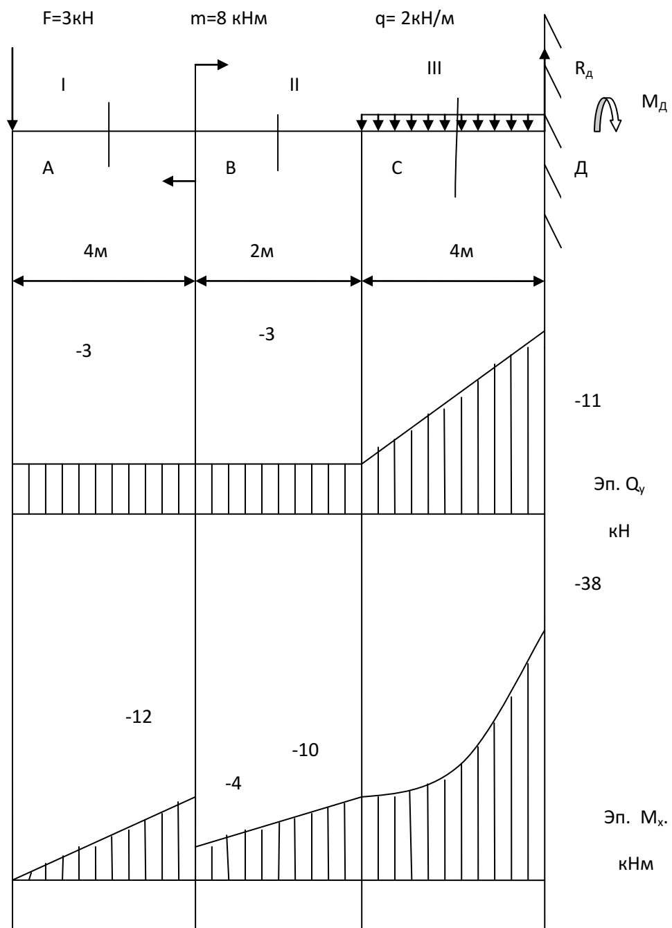
Рисунок 2.- Эпюры внутренних силовых факторов при изгибе балки.
