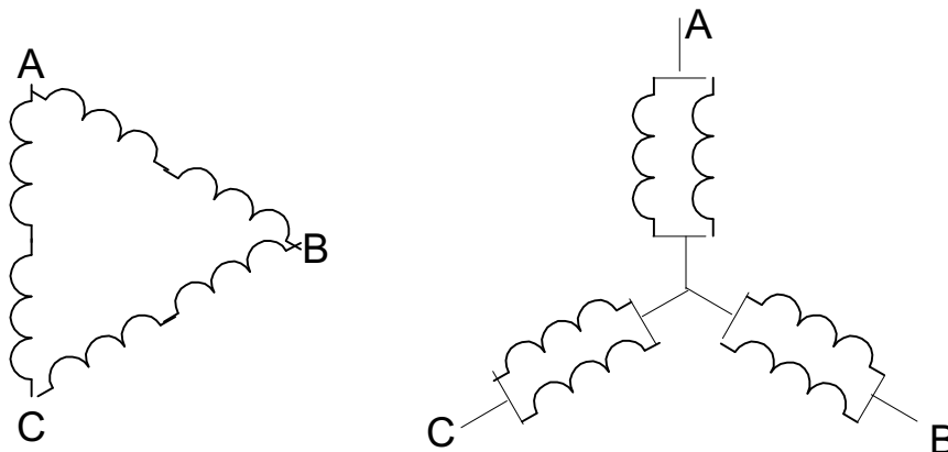
Рис.16.4. Двухскоростной АЭД со схемой \Delta/Y . (Треугольник -двойная звезда). Таблица 16.4. Частоты вращения многоскоростного АЭД с короткозамкнутым ротором.
