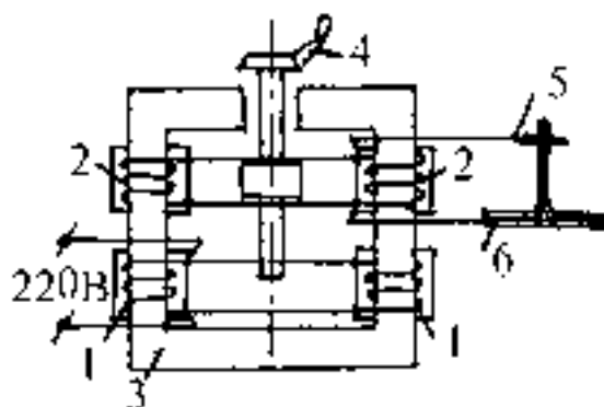
Рисунок 11.5. Принцип работы сварочного трансформатора
