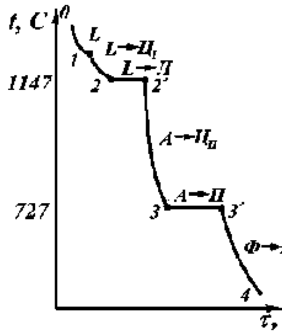
Рисунок 3.6. Сплав 4 (заэвтектический чугун)
