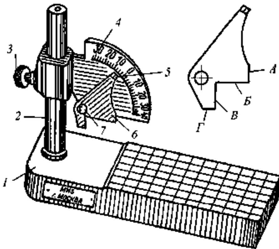
Рисунок 13.3. Настольный угломер
