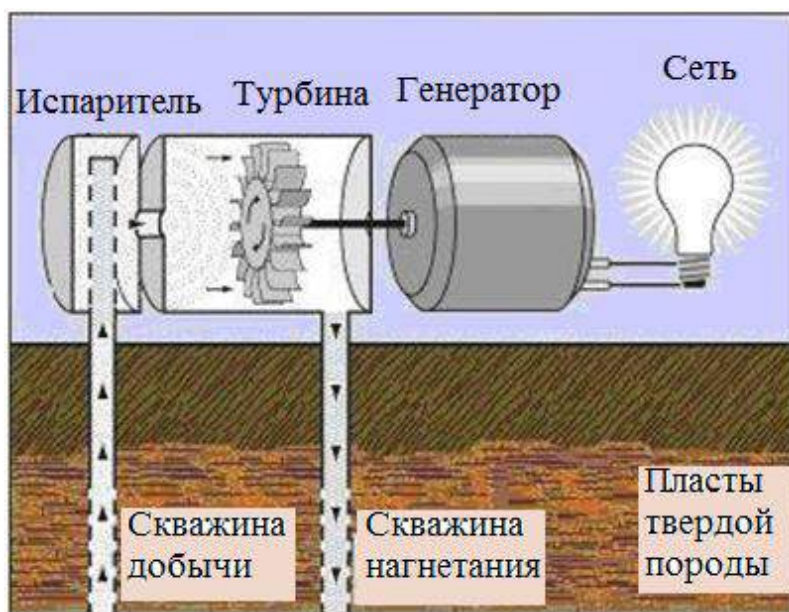
Рисунок 2 - Принцип работы геотермальной электростанции с непрямым типом производства энергии
