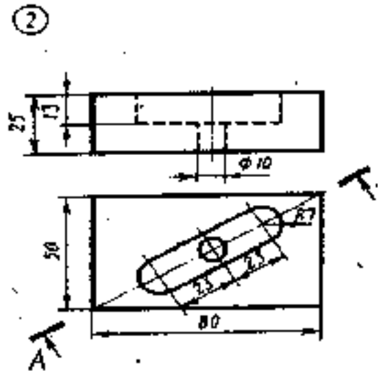
Плита
