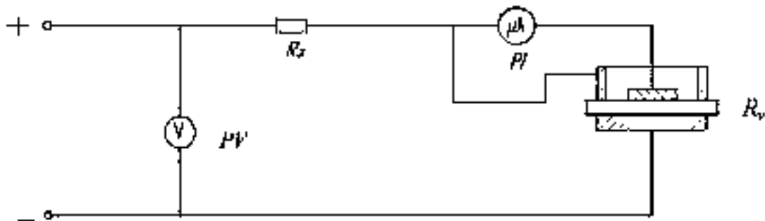
Рисунок 20.1. Схема для измерения объемного сопротивления
