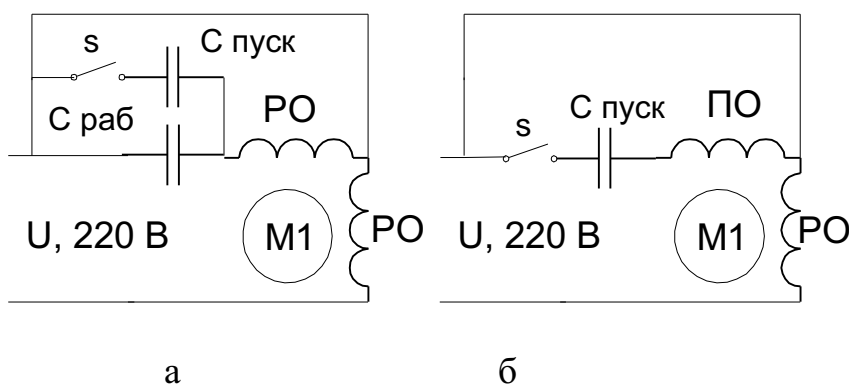
Рис.22.2. Схема включения однофазного электродвигателя.
