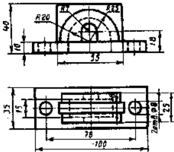
Крышка
