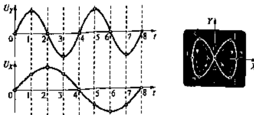
Рис. 3. Метод фигур Лиссажу
