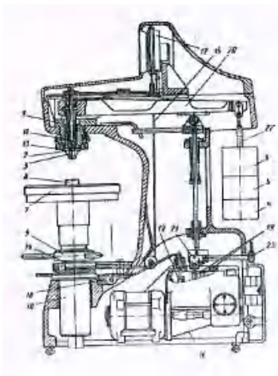
Рисунок 2.4 Схема прибора ТК-2 (типа Роквелла)
