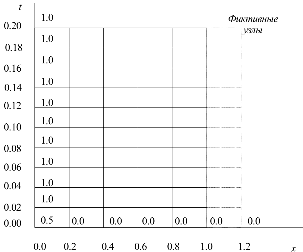
Рис. 3.5. Двумерная сетка с граничными и начальными условиями
