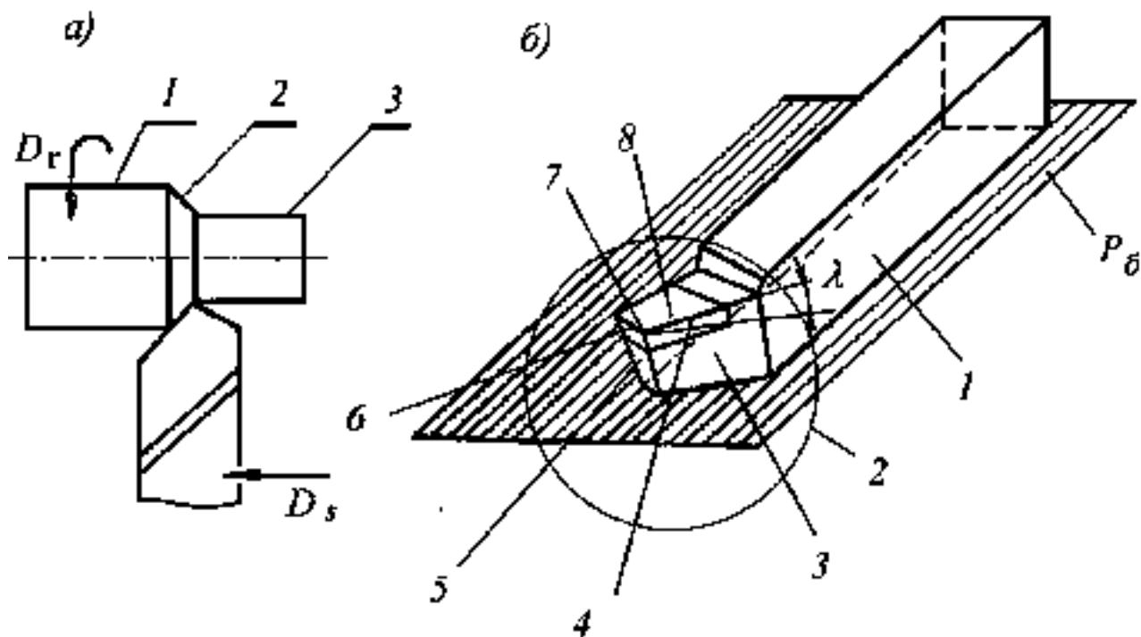
Рисунок 13.1. Схема точения (а), токарный проходной резец (б)
