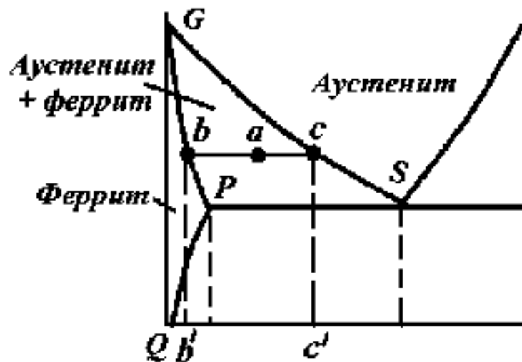
Рисунок 3.2. Диаграмма состояния
