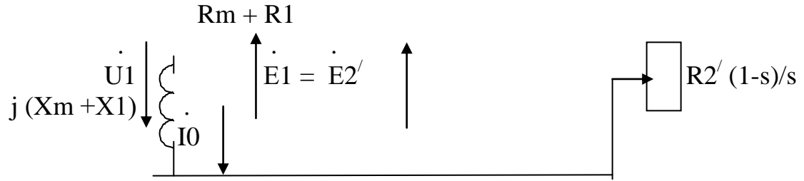
Рис.15.1. Эквивалентная схема одной фазы АЭД.
