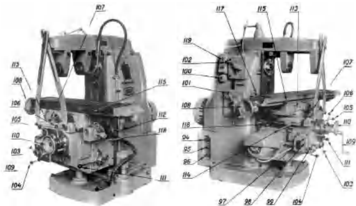
Рисунок 16.2. Расположение органов управления фрезерным станком модели 6Н81Г
