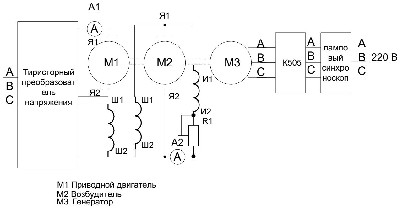
Рис. 13.2. Схема СГ, синхронизированного с сетью.
