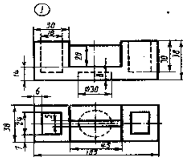
Опора
