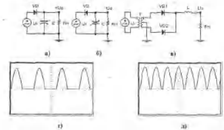
Рис. 1. Одно- (а, б) и двухполупериодный (в) выпрямители и осциллограммы сигналов при активной нагрузке (г, д)
