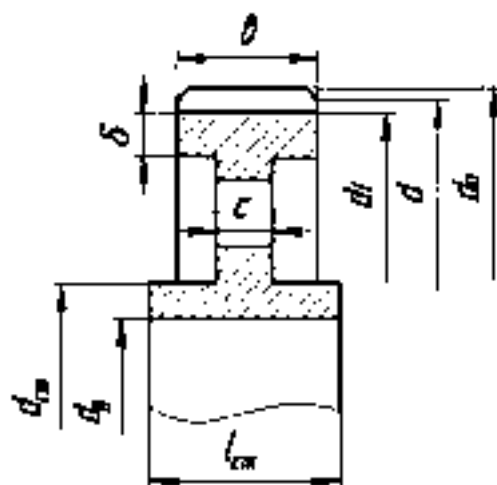
Рис. 2 Эскиз шестерни (колеса).
