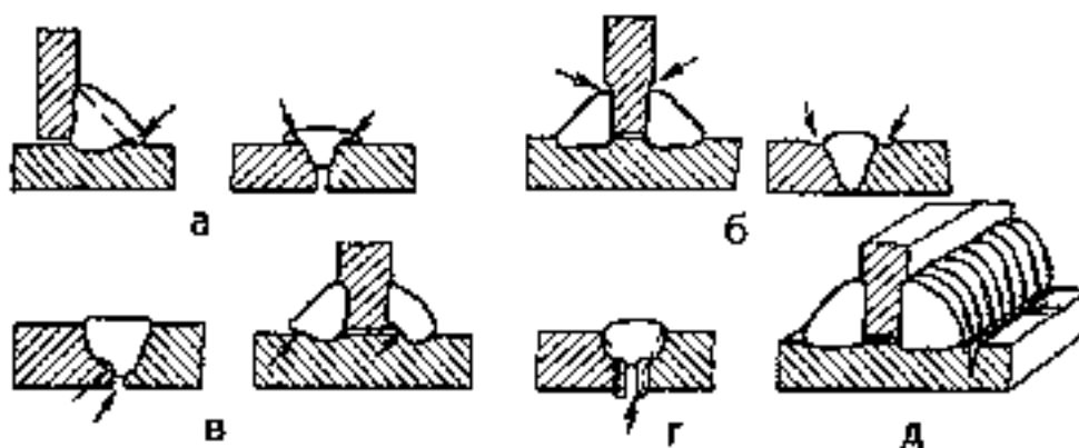
Рисунок 11.9. Наружные дефекты сварного шва:
