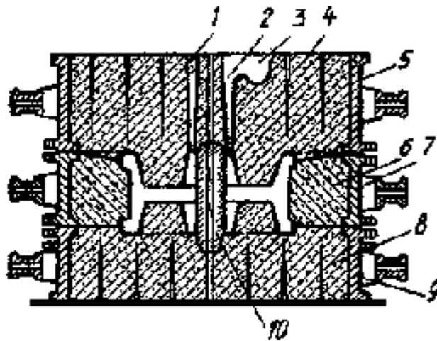
Рисунок 10.2. Форма для отливки шкива, изготовленная в трех опоках: 1 — выпор, 2 — стояк, 3 — литниковая чаша. 4 — верхняя часть формы, 5 — верхняя опока, 6 — средняя часть формы, 7 — средняя опока, 8 — нижняя часть формы, 9 — нижняя опока, 10 — стержень
