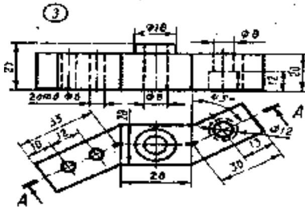
Крышка
