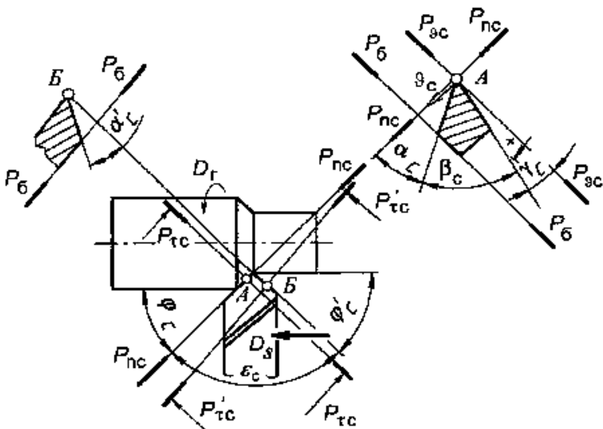
Рисунок 13.2. Углы токарного проходного резца
