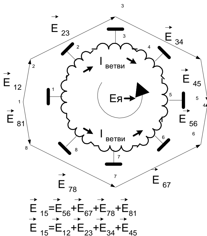
Рис.18.6. Распределение ЭДС в соответствии с потенциальной кривой. Точки 1,2,...8- контакты коллектора.
