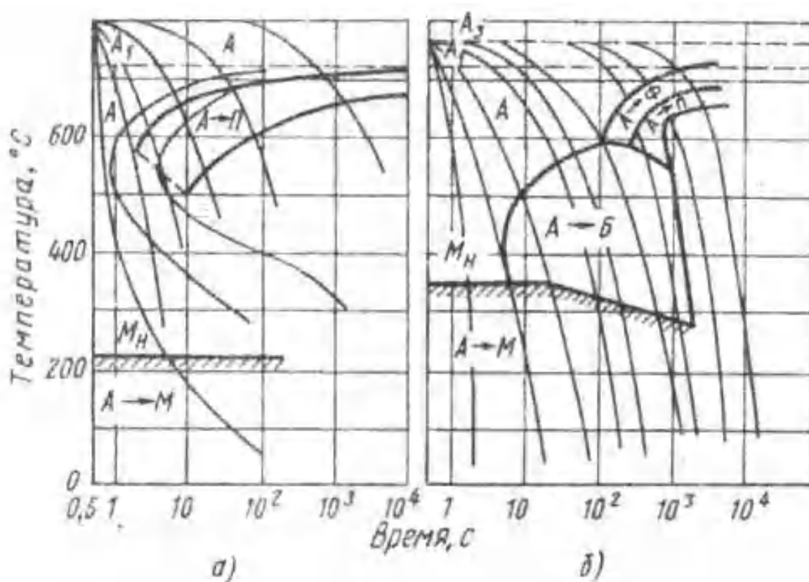
Рисунок 8.9. Термокинетические диаграммы превращения переохлажденного аустенита
