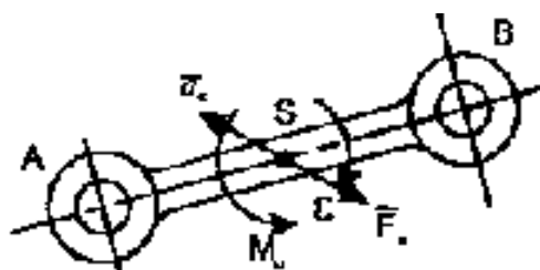
Рис. 22 Сила и момент инерции звена плоского механизма
