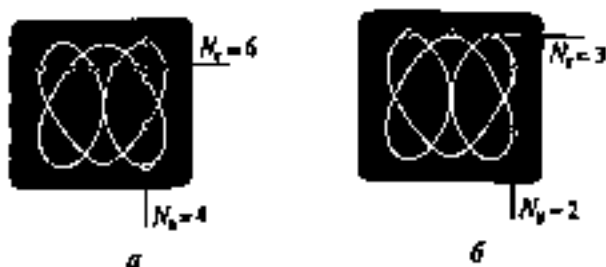
Рис. 4. Определение точек пересечения (а) или касания (б)
