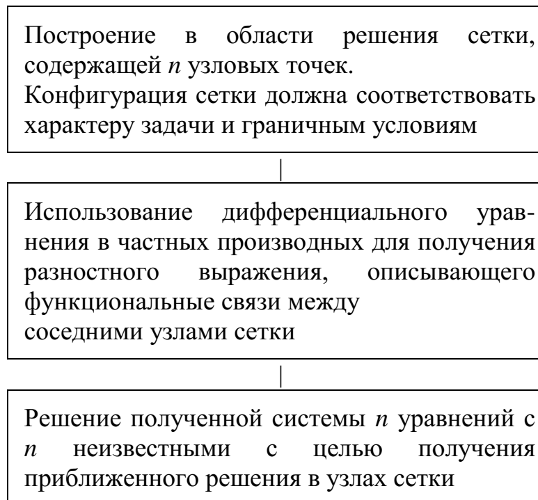
Рис. 3.1. Основные этапы численного решения дифференциальных уравнений
