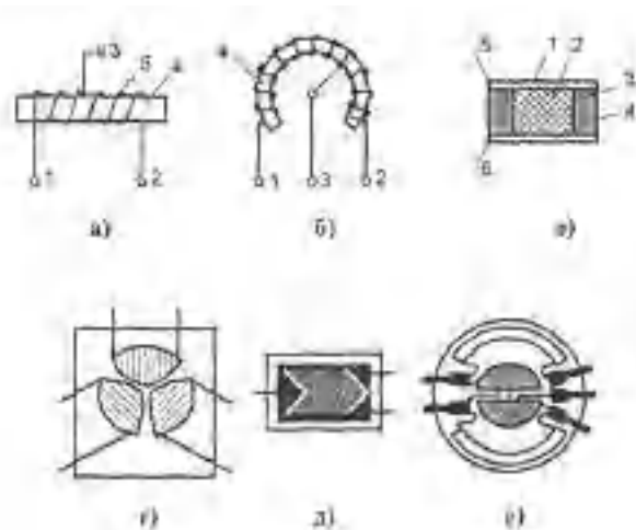
Рис. 1. Конструктивные схемы реостатных ИП(а, б), ИП контактного сопротивления (в) и тензометрических ИП(г, д, е)
