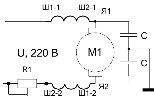
Рис.22.3. Схема включения однофазного коллекторного электродвигателя.
