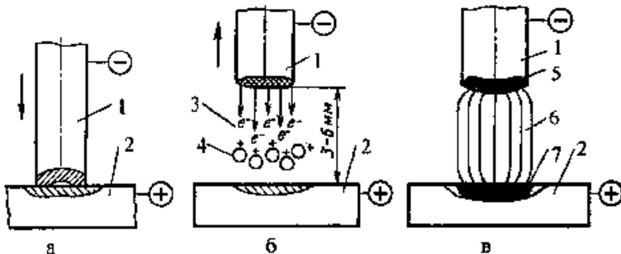
Рисунок 11.3. Схема процесса зажигания дуги
