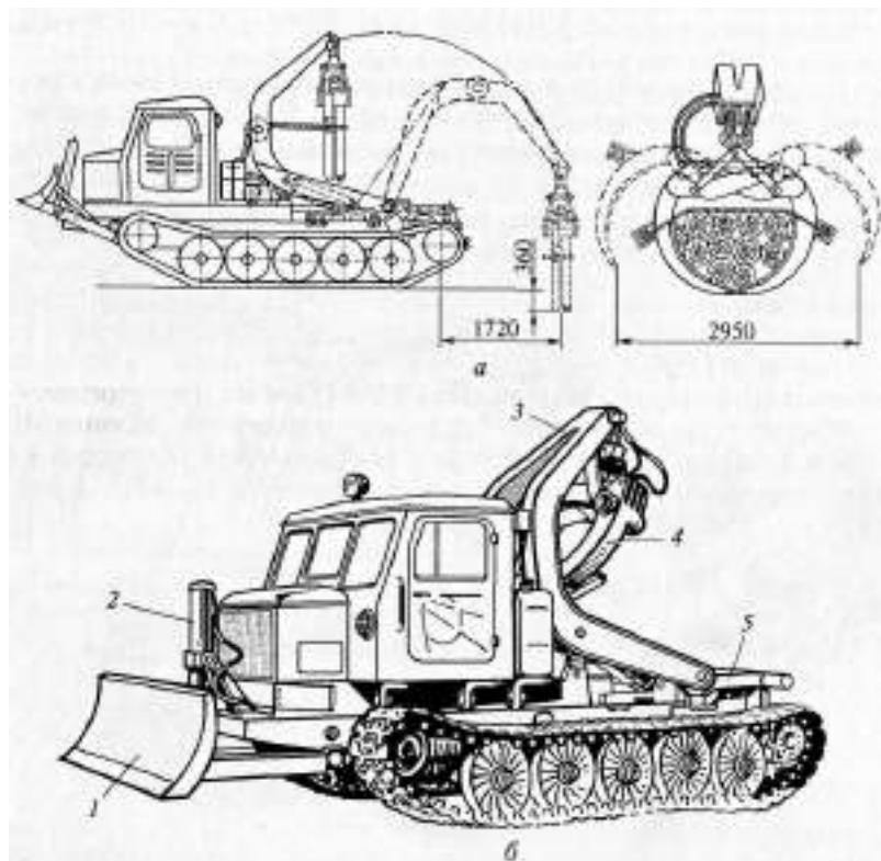
Рис. 7. Технологическое оборудование трактора ЛТ-154: a — схема работы; b — общий вид; 1 — толкатель; 2 — гидроцилиндр; 3 — стрела; 4 — клещевой пачковый захват; 5 — щит
