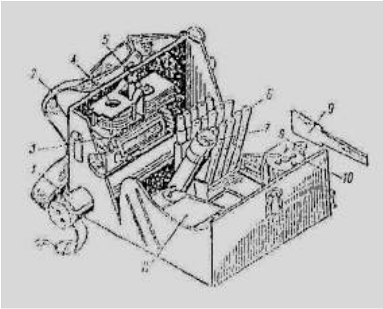
Рис. 4. Воинский прибор химической разведки
