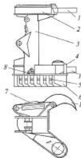
Рис. 3.5. Захватно-срезающее устройство: 1 — зажимные крюки; 2, 4 — соответственно верхняя и нижняя призмы; 3 — стойка; 5 — механизм срезающего; 6 — рама пилы; 7 — гидроцилиндр; 8 — трубопровод
