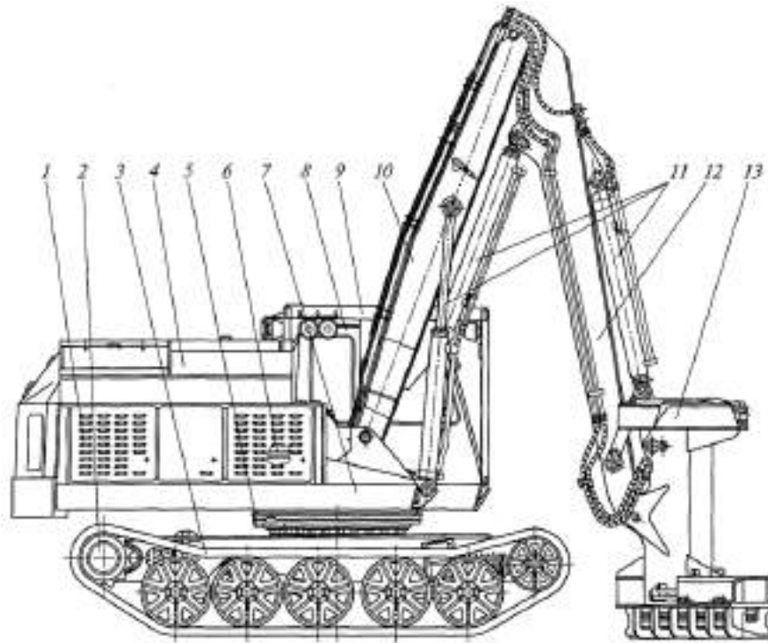
Рис. 3.4. Валочно-палетирующая машина МЛ-119А:
