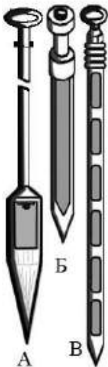
Рисунок 11 - Щупы: а - конусный; б - мешочный; в – цилиндрический
