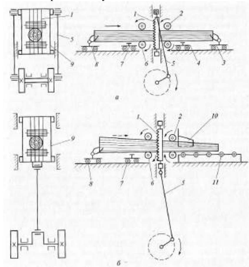
Рис. 6. Схемы двухшатунной (а) и одноштанной (б) лесопильных рам:
