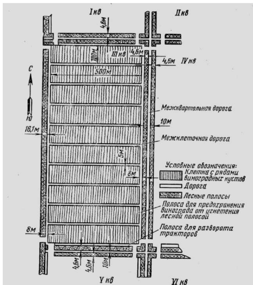
Рисунок 5. Схема организации территории под виноградник на ровном месте без орошения
