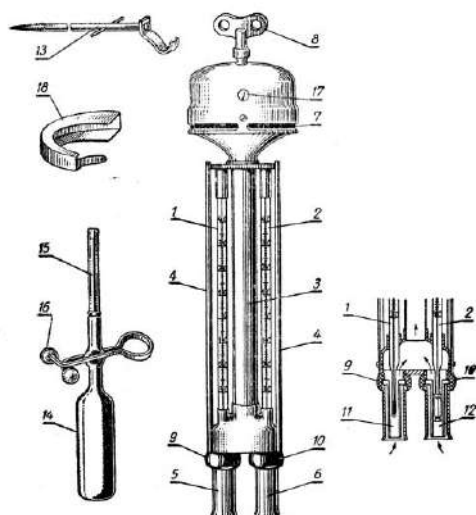
Рис. 12 Аспирационный психрометр
