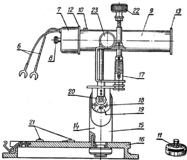
Термоэлектрический актинометр
