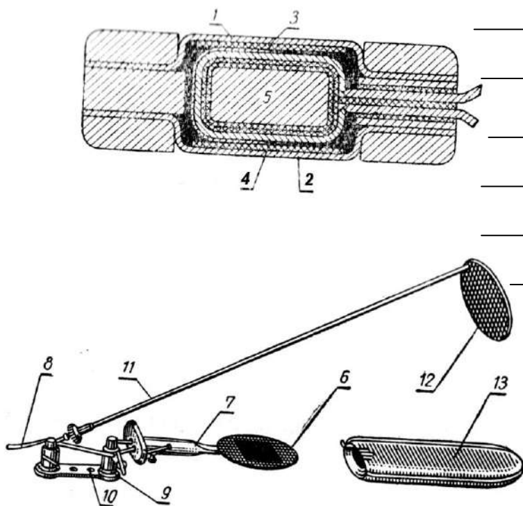
Термоэлектрический балансомер
