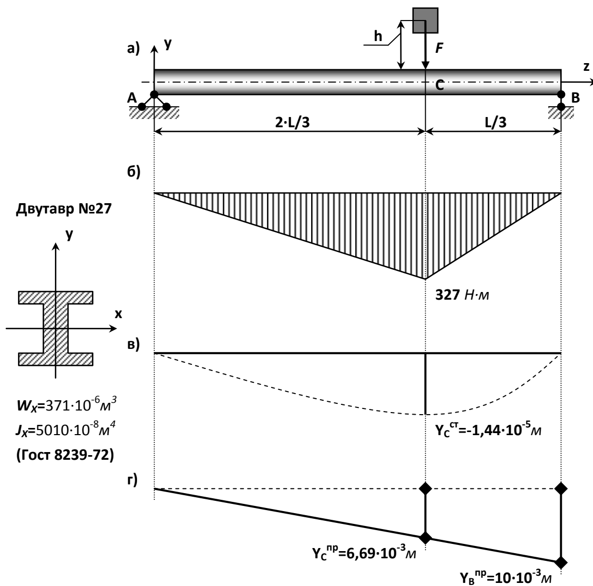
а) схема нагружения; б) эпюра M , кН·м; в) эпюра прогиба на жесткой опоре B;
