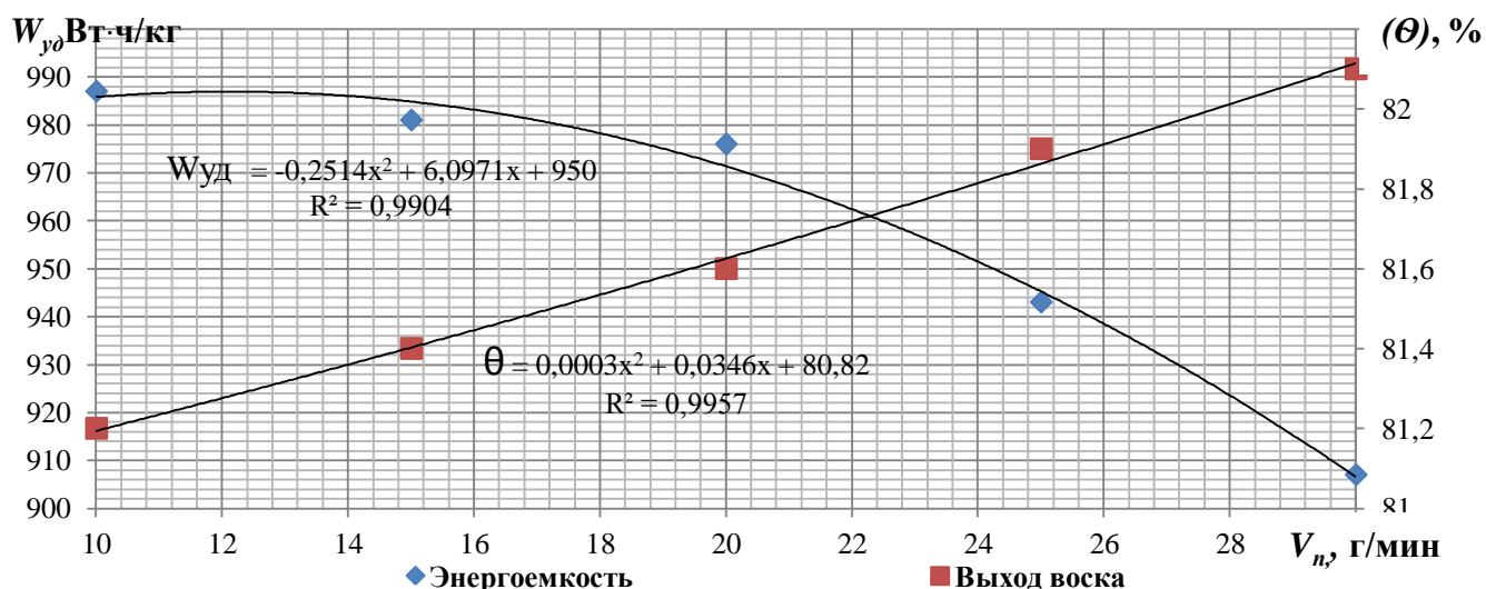
Рисунок 7 – Изменение энергоёмкости процесса вытопки ( W_{уд} ) и выхода воска ( \theta ) от подачи пара ( V_n )
