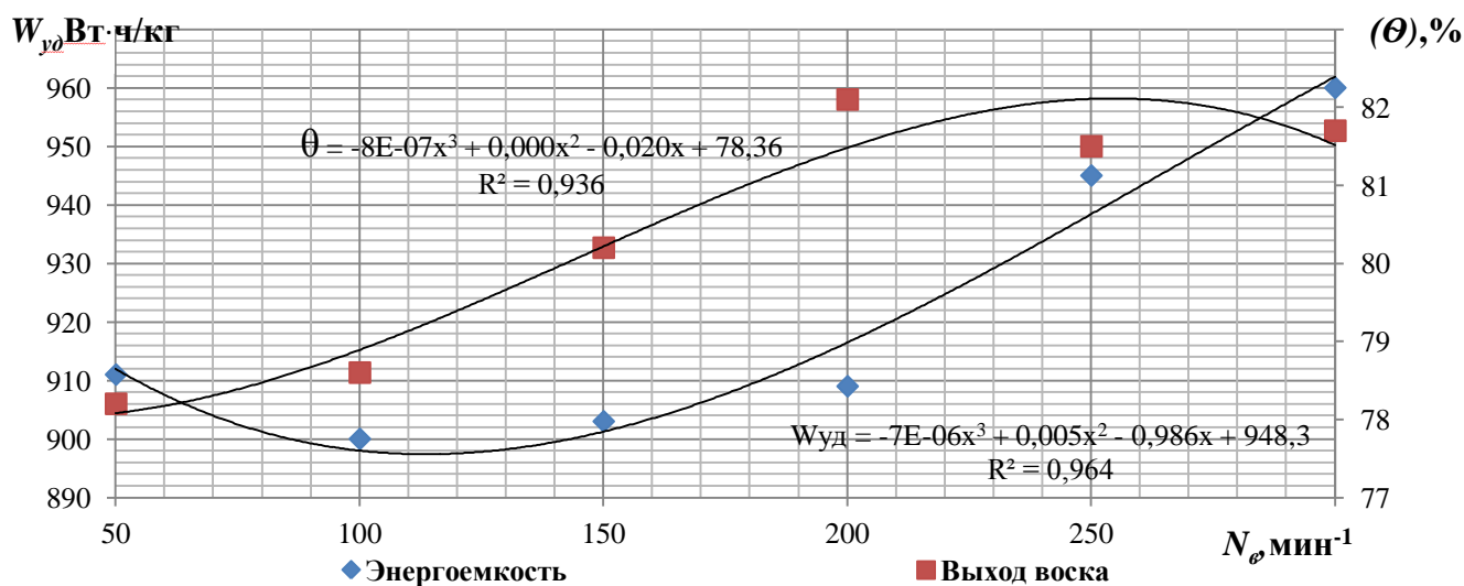
Рисунок 6 – Изменение энергоёмкости процесса вытопки ( W_{уд} ) и выхода воска ( \theta ) от частоты вращения шнека воскопресса ( N_{ш} )
