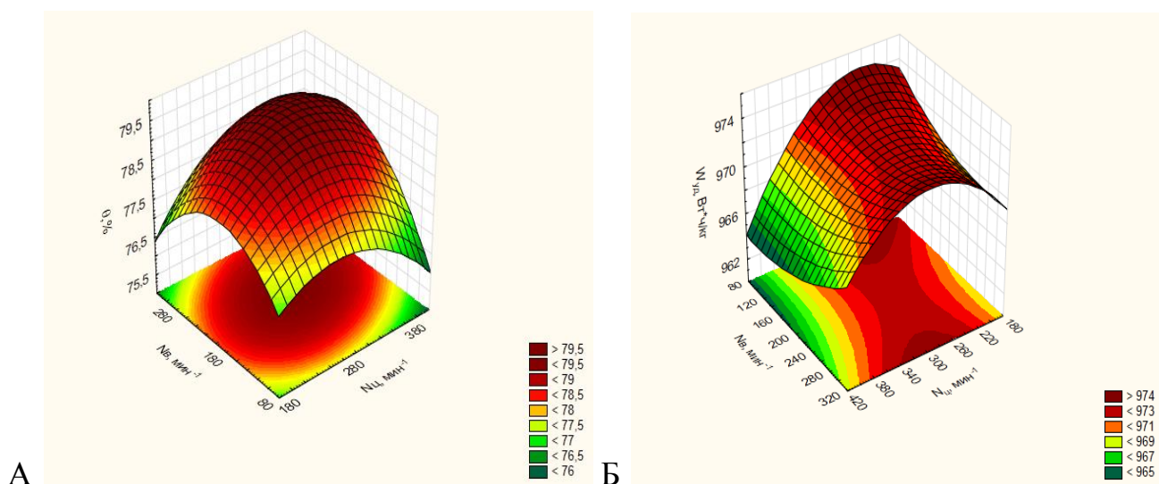
Рисунок 8 – Поверхности отклика, характеризующая выход воска (А) и энергоёмкости (Б) от частоты вращения ротора центрифуги N_{ц} и частоты вращения шнека воскопресса N_{ш} при расходе пара V_n=30 г/мин
