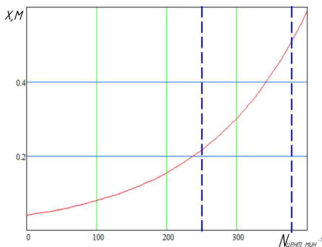
Рисунок 3 — Зависимость перемещения (x) капли воска от частоты вращения ротора центрифуги ( N_{цент} )
