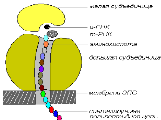
Строение рибосомы
