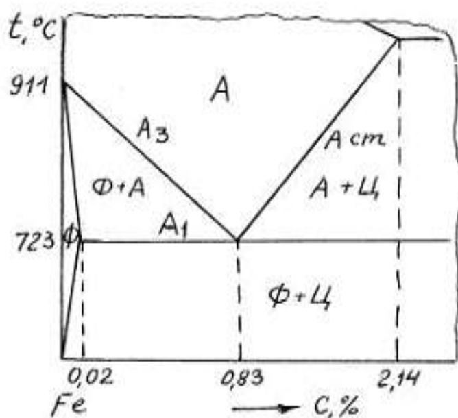
Рисунок 1. Фрагмент диаграммы Fe – C с указанием фаз и критических температур (A1, A2, Ast)
