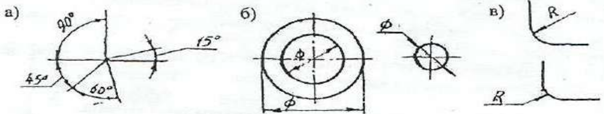
Рисунок 7.4 – Нанесение размеров дуг, диаметров и радиусов
