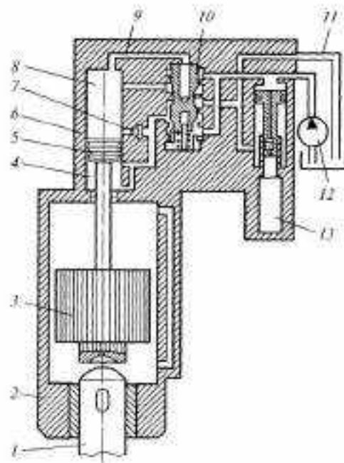
Рисунок 15. Принципиальная схема гидромолота с гидроаккумулятором
