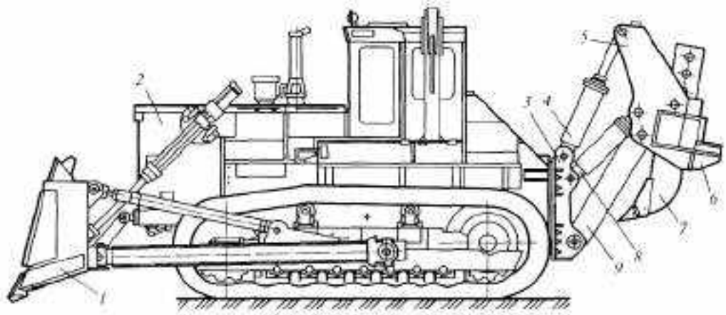
Рис. 4.13. Бульдозер-рыхлитель на базе трактора Т-35.01: 1 – бульдозерное оборудование (полусферический отвал); 2 – трактор; 3 – опорный кронштейн; 4 – гидродлиндр регулирования угла рыхления; 5 – рабочая балка; 6 – буферное устройство; 7 – зуб; 8 – гидродлиндр поворота – отклонения рыхлителя; 9 – нижняя тяга
