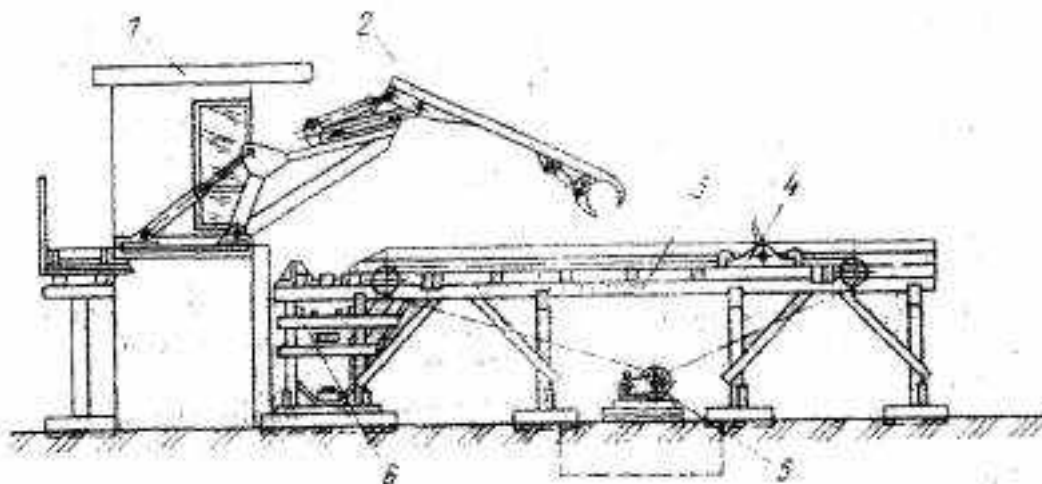
Рис. 1. Схема размещения манипулятора ЛО-13С и разгрузочно-растаскивающего устройства РРУ-10М:
