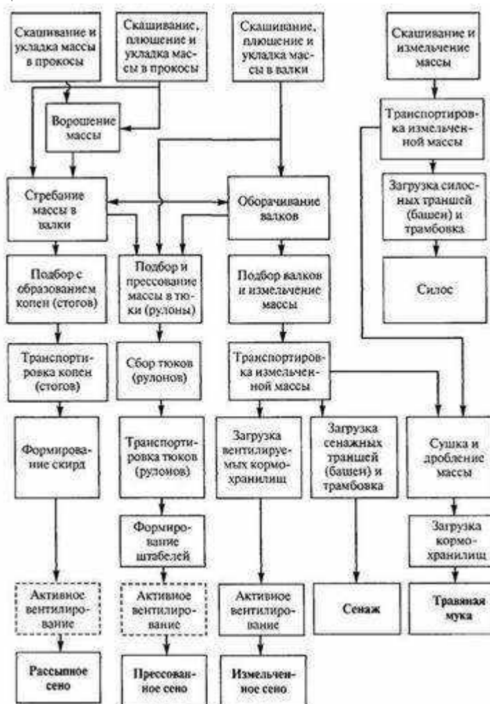
Рис.1.Схема технологий
