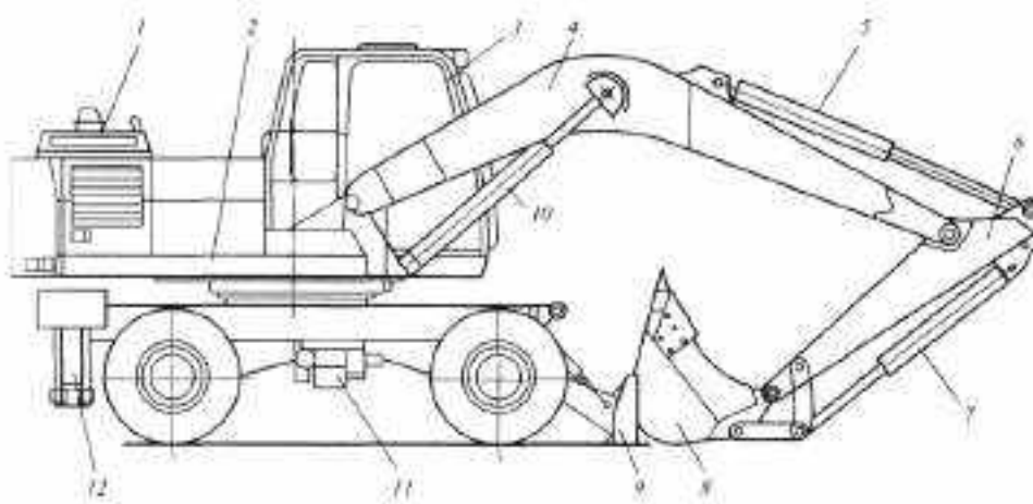
Рисунок 18. Одноковшовый полноповоротный пневмоколесный экскаватор ЕК-18:
