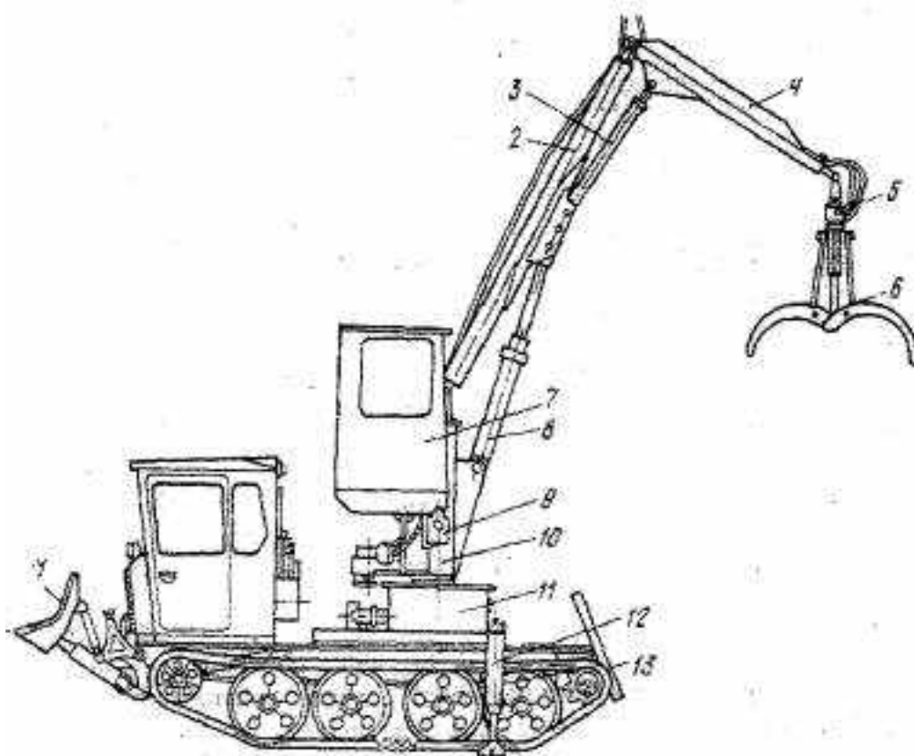
Рис. 4. Погрузчик-штабелер ПШ-80:
