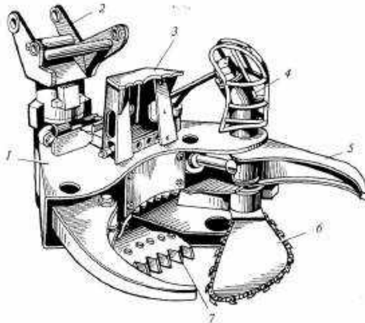
Рис. 3.8. Захватно-срезающее валочное устройство машины ЛП-17: 1 — корпус; 2 — подвеска; 3 — опорная призма; 4 — гидромотор привода пилы; 5 — захват; 6 — пила; 7 — гидродомкрат
