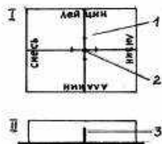
Рис. 3. Хроматография аминокислот: I) общий вид радиальной хроматограммы; II) схема хроматографической камеры
