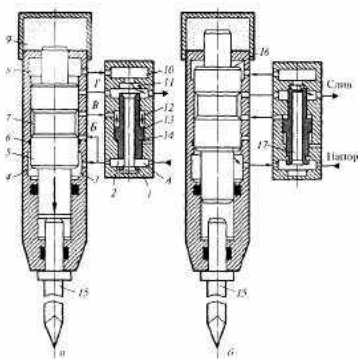
Рисунок 16. Принципиальная схема гидропневматического молота
