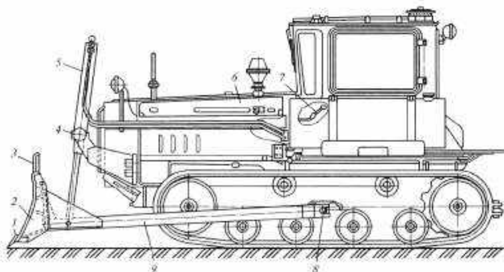
Рис. 4.9. Бульдозер Д3-42Т
