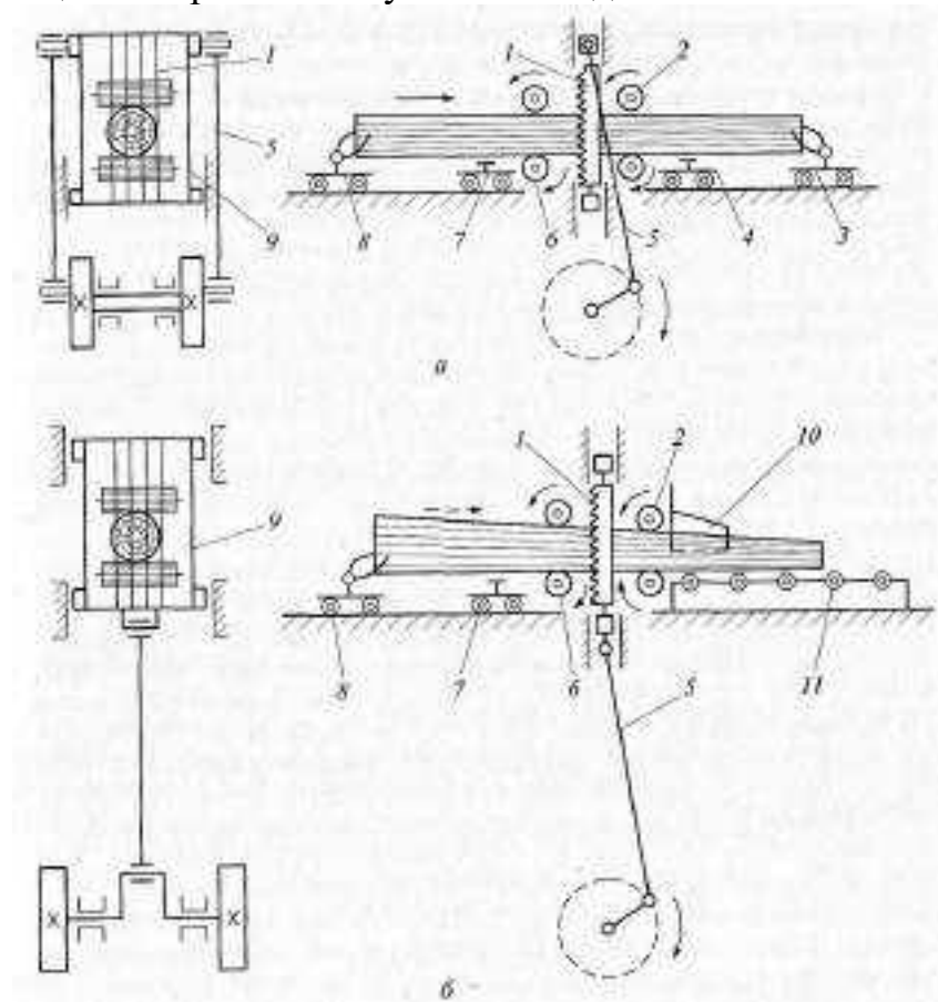
Рис. 6. Схемы двухштанной (а) и одноштанной (б) лесопильных рам: 1 — пилы; 2, 6 — подающие валцы; 3, 4, 7, 8 — тележки; 5 — кривошипно-шатунный механизм; 9 — пильная рамка; 10 — направляющий нож; 11 — рольганг
