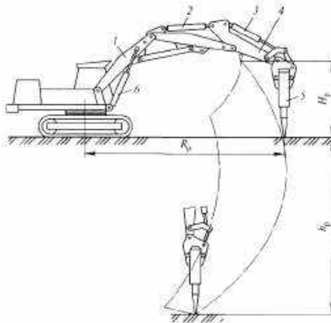
Рисунок 14. Экскаватор, оборудованный гидравлическим молотом
