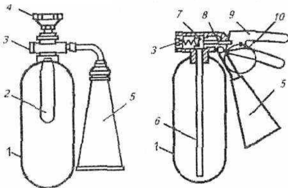
Схема огнетушителя ОУ-2
