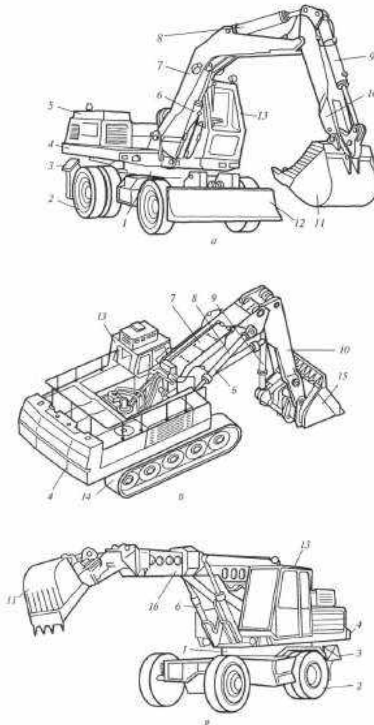
Рисунок 7. - Одноковшовые гидравлические полноповоротные экскаваторы с жесткой подвеской рабочего оборудования:
