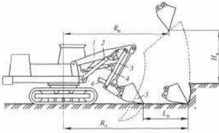
Рисунок 11. Экскаватор с погрузочным оборудованием
