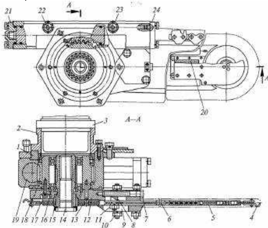
Рис. 3.6. Механизм срезания:
