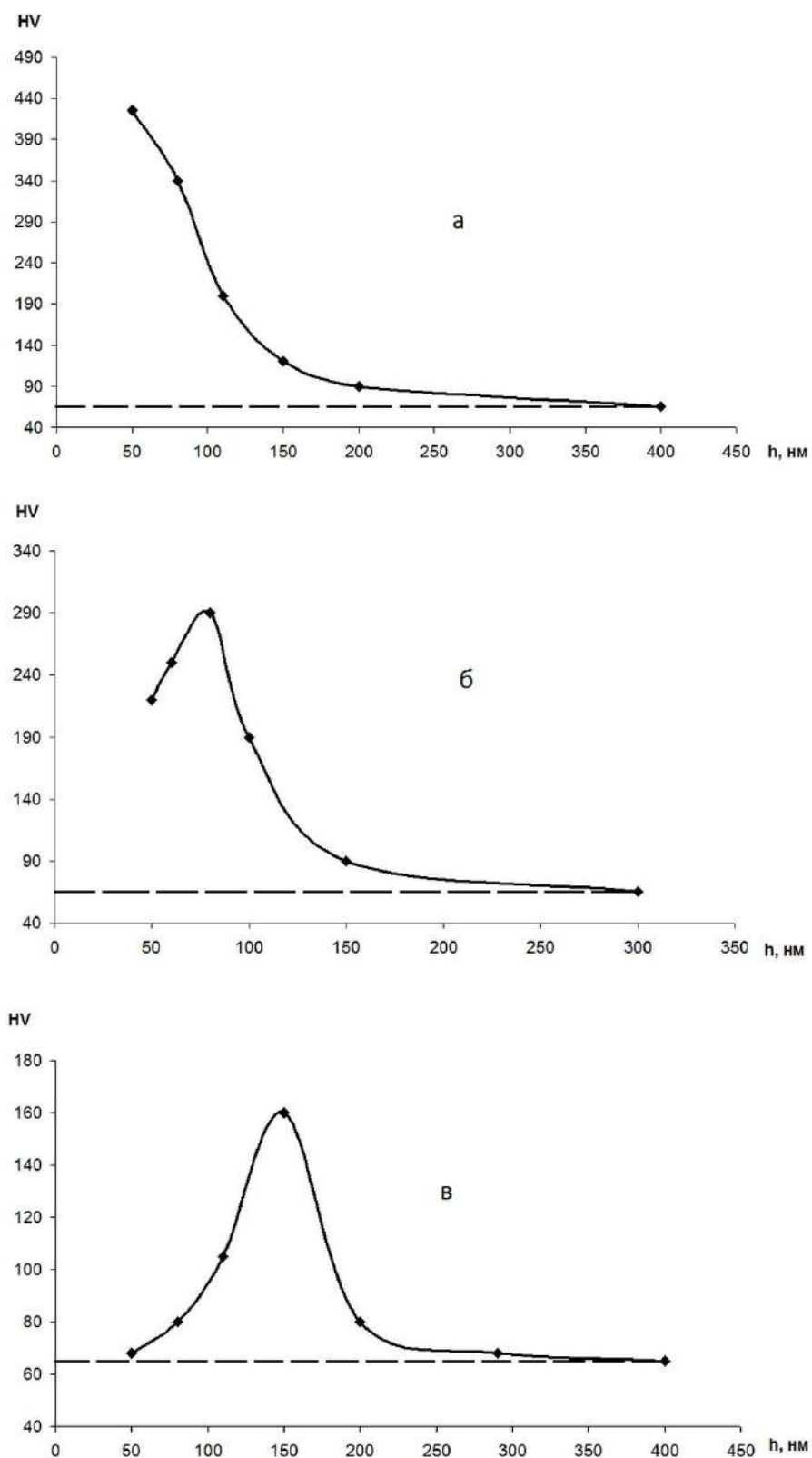
Рисунок 3 -Твердость нанопокровтий в зависимости от их толщины. Покровтие: золото; основа: а – вольфрам, б – никель, в – железо.
