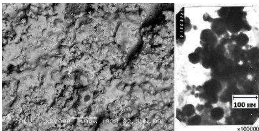
Рисунок 3 -Наноструктурированное покрытие на основе твердого сплава с износостойкой керамической матрицей ( \text{WC-Al}_2\text{O}_3 ). Размер зерна 5-50 нм.
