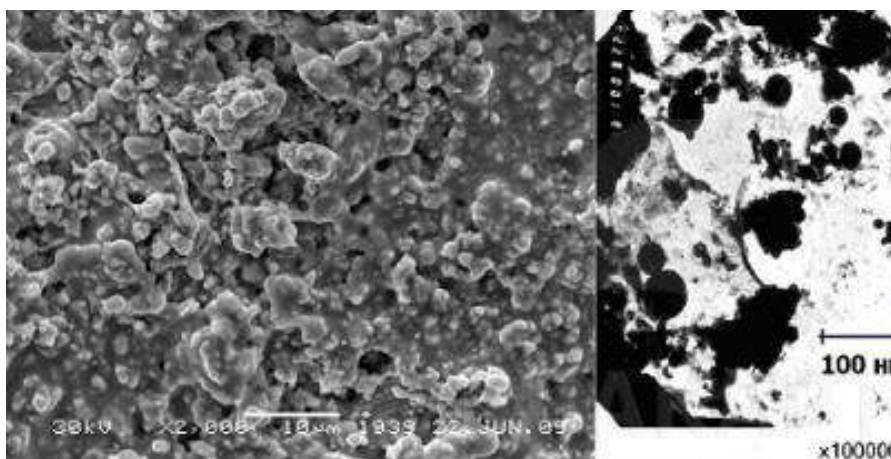
Рисунок 2 -Наноструктурированное покрытие на основе твердого сплава с антифрикционной керамической матрицей ( \text{WC-TiO}_2 ). Размер зерна 10-50 нм.
