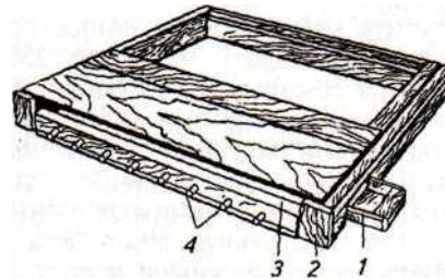
Рис.6. Магазинный пыльцеуловитель:
