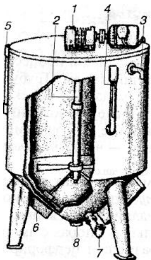
Рис. 51. Медоотстойник:
