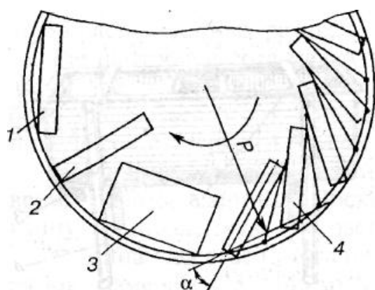
Рис.48. Схема расположения рамок в роторе медогонки:
