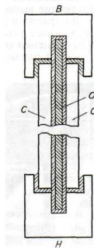
Рис. 13. Детали устройства ядоприемной рамки:
