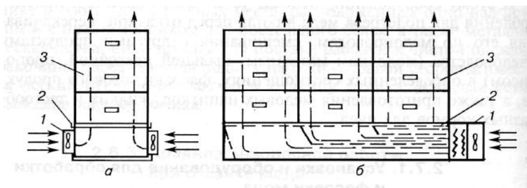
Рис. 52. Схема электрокалориферной установки для подогрева корпусов с медовыми сотами перед откачкой:
