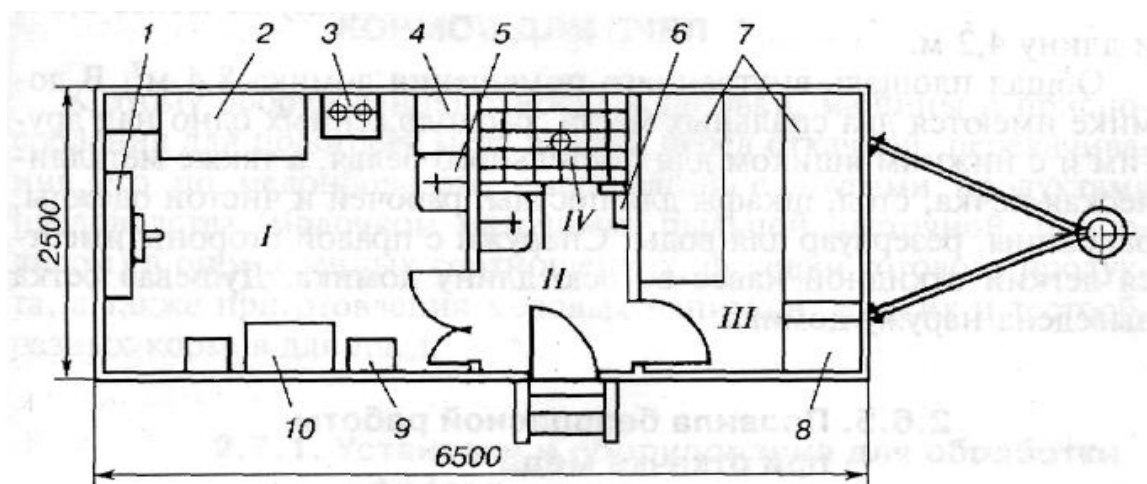
Рис. 51. Вагон пчеловодный:
