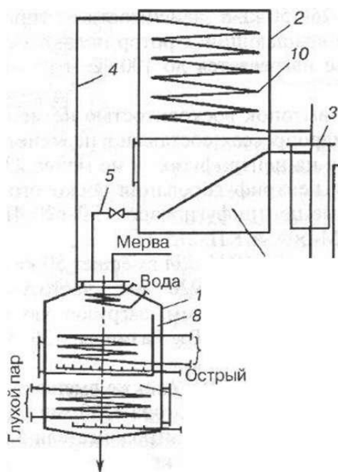
Рис.55. Схема устройства воскоэкстракционного аппарата АВ-171:
